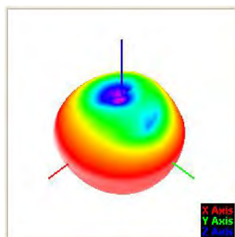
700MHz
