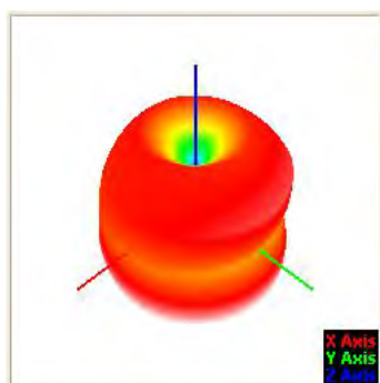
2690MHz
