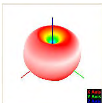
3300MHz
