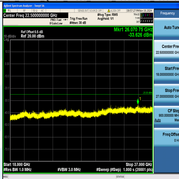
Band7_20MHz_QPSK_21350_1RB#0_18000~27000_18000~27000
