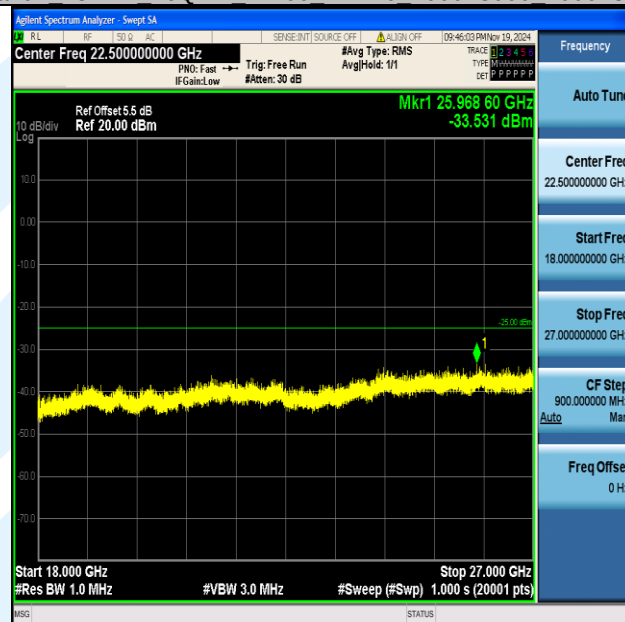
Band7_15MHz_16QAM_21100_1RB#0_18000~27000_18000~27000
