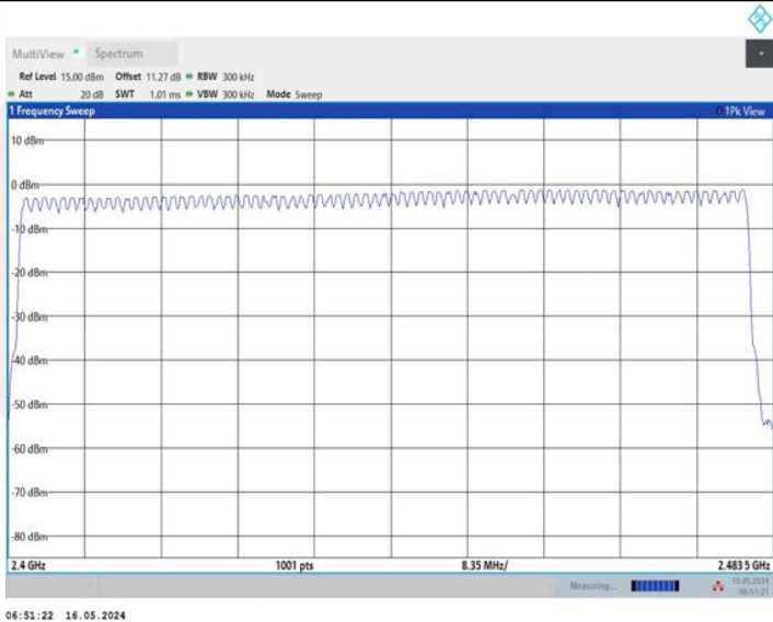
3DH5_Ant1_Hop
