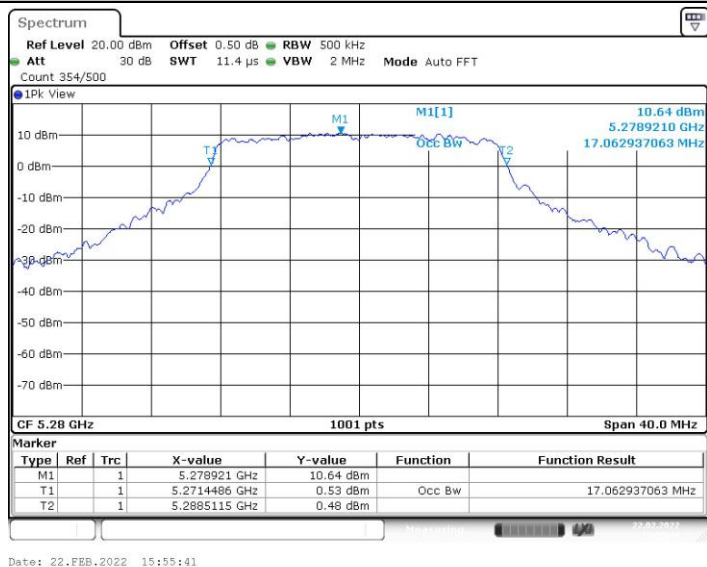
11A_Ant9_5280
