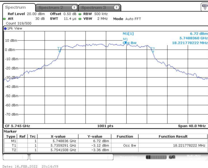
11N20MIMO_Ant9_5745
