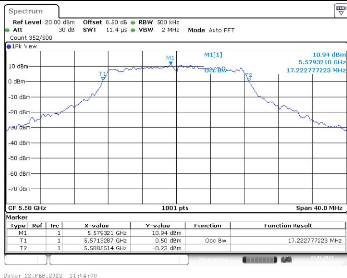
11A_Ant8_5580
