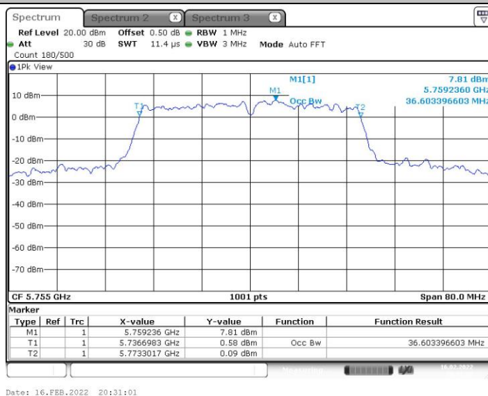
11N40MIMO_Ant9_5755
