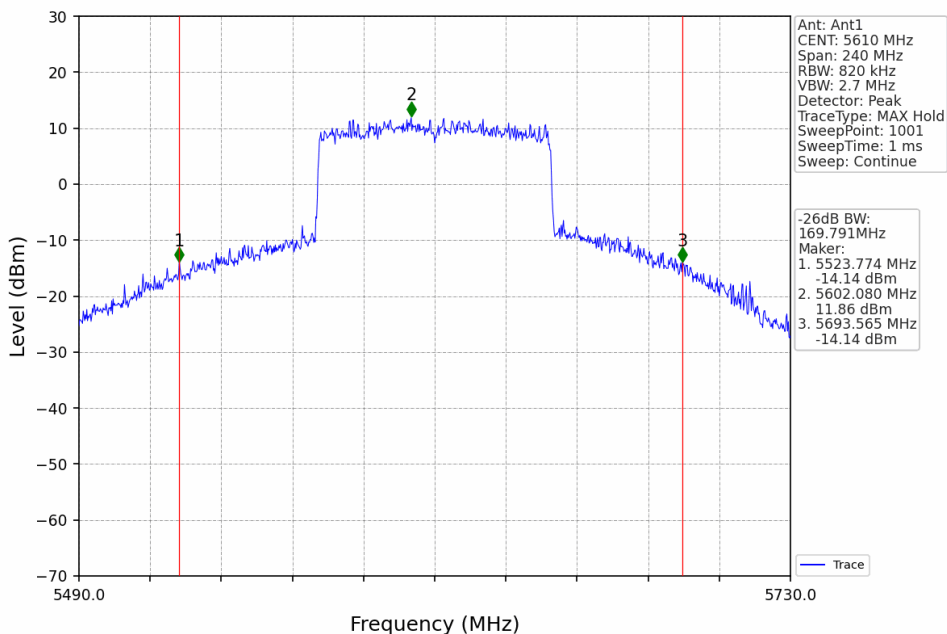
802.11ax(HEW80)_HCH_5610MHz_RU996_Left_Ant1_NTNV
