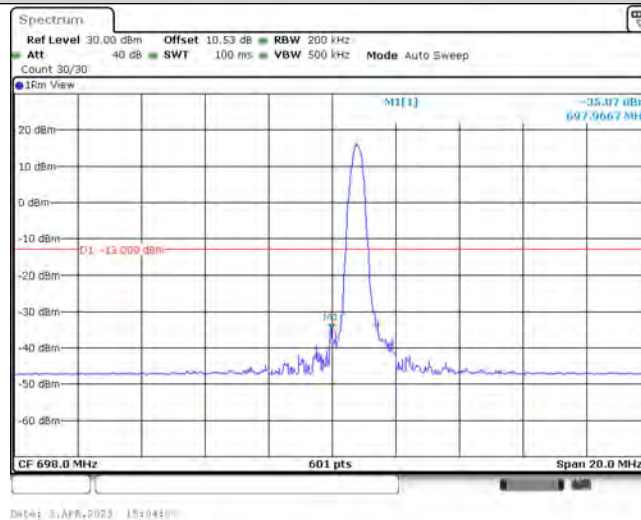
Band85-10MHz-16QAM-134052-1-0-Low--35.07-PASS
