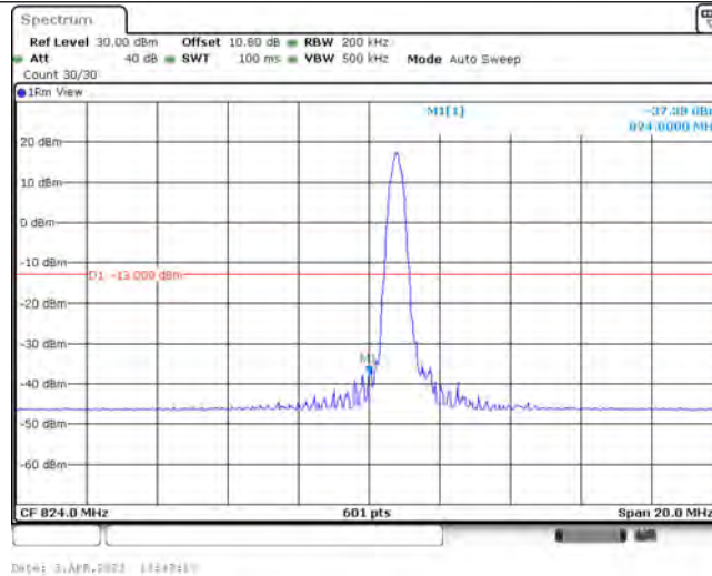
Band26-10MHz-16QAM-26840-1-0-Low--37.38-PASS
