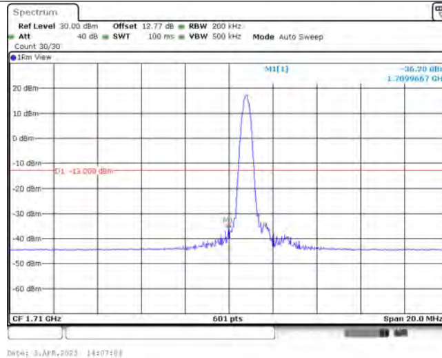
Band4-10MHz-16QAM-20000-1-0-Low--36.20-PASS
