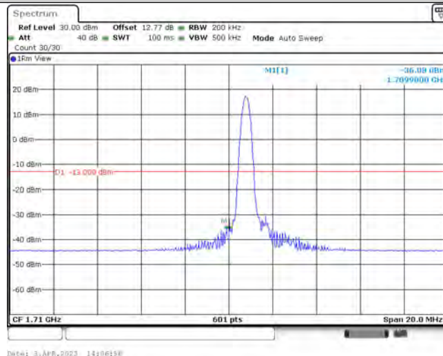
Band4-10MHz-QPSK-20000-1-0-Low--36.08-PASS
