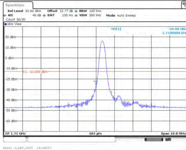
Band66-5MHz-16QAM-131997-1-0-Low--26.08-PASS
