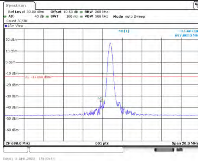
Band85-10MHz-QPSK-134052-1-0-Low--35.66-PASS
