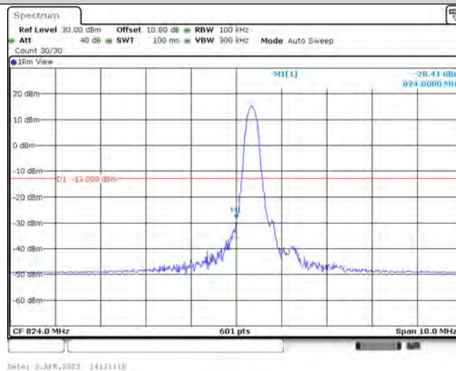
Band5-5MHz-16QAM-20425-1-0-Low--28.41-PASS
