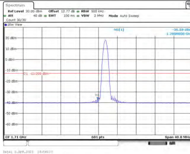
Band66-20MHz-16QAM-132072-1-0-Low--36.58-PASS
