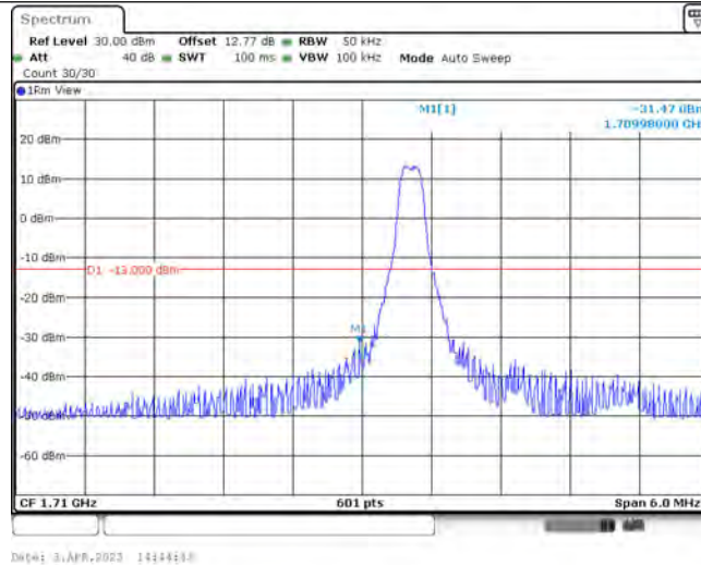
Band66-3MHz-QPSK-131987-1-0-Low--31.47-PASS
