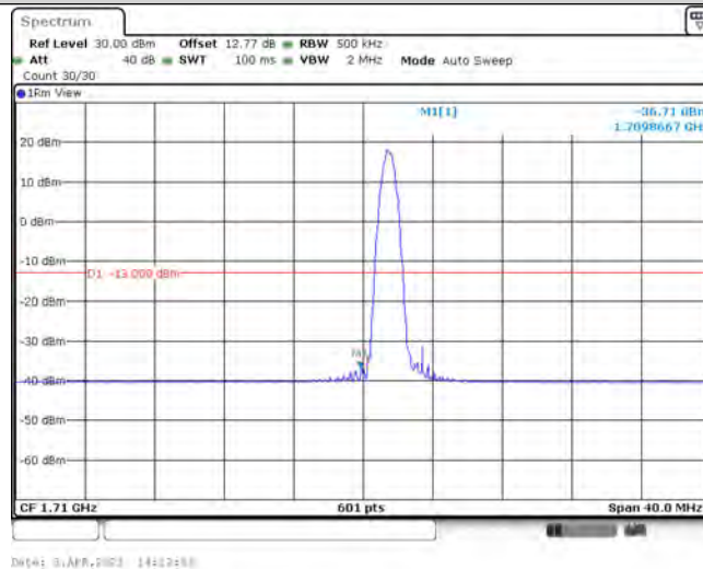
Band4-20MHz-16QAM-20050-1-0-Low--36.71-PASS
