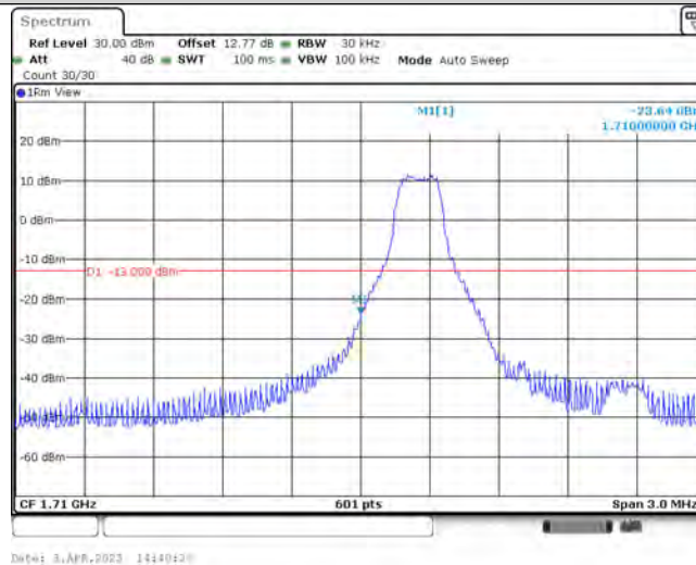
Band66-1.4MHz-QPSK-131979-1-0-Low--23.64-PASS
