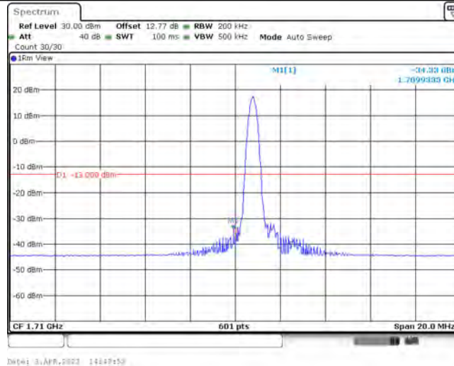
Band66-10MHz-QPSK-132022-1-0-Low--34.33-PASS
