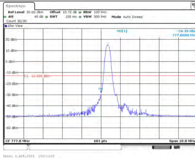
Band13-5MHz-16QAM-23205-1-0-Low--28.18-PASS
