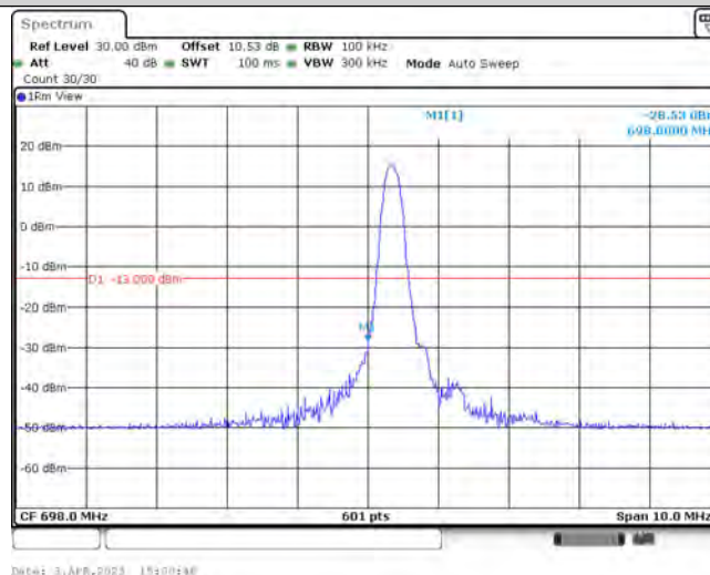
Band85-5MHz-16QAM-134027-1-0-Low--28.53-PASS
