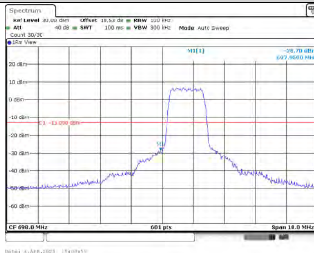
Band85-5MHz-QPSK-134027-6-0-Low--28.70-PASS
