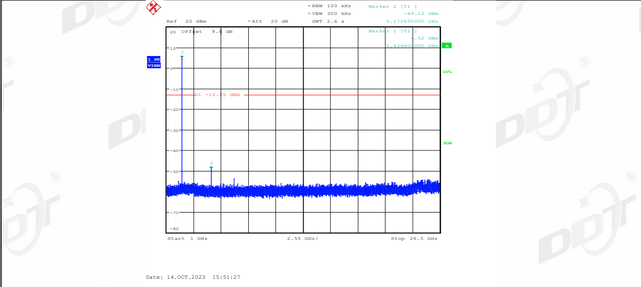
GFSK 2M Ant1_2478_0~Reference
