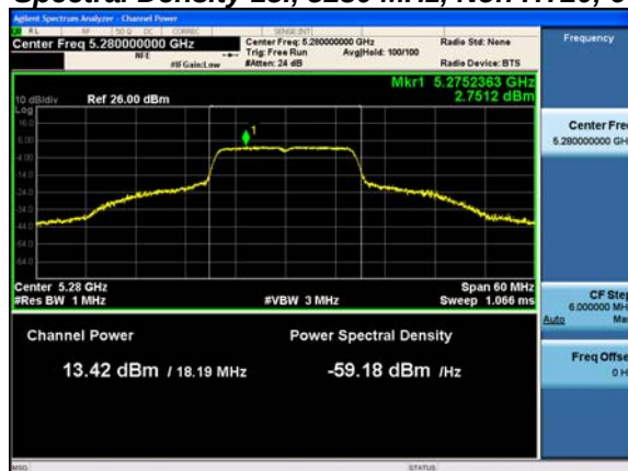
Antenna A
