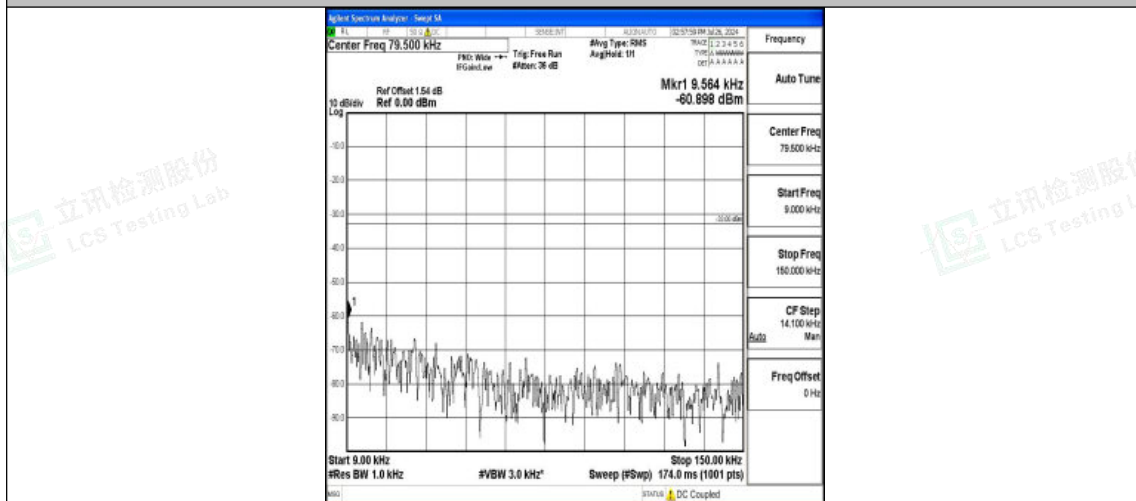
Band5-3MHz-QPSK-20635-1RB#0-0.009~0.15-PASS
