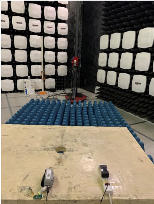
3GHz – 18GHz
