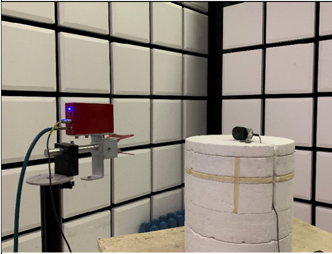
18GHz – 26GHz
