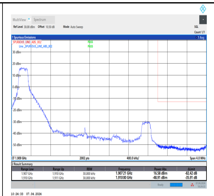
Band2_3MHz_QPSK_19185_1RB#0
