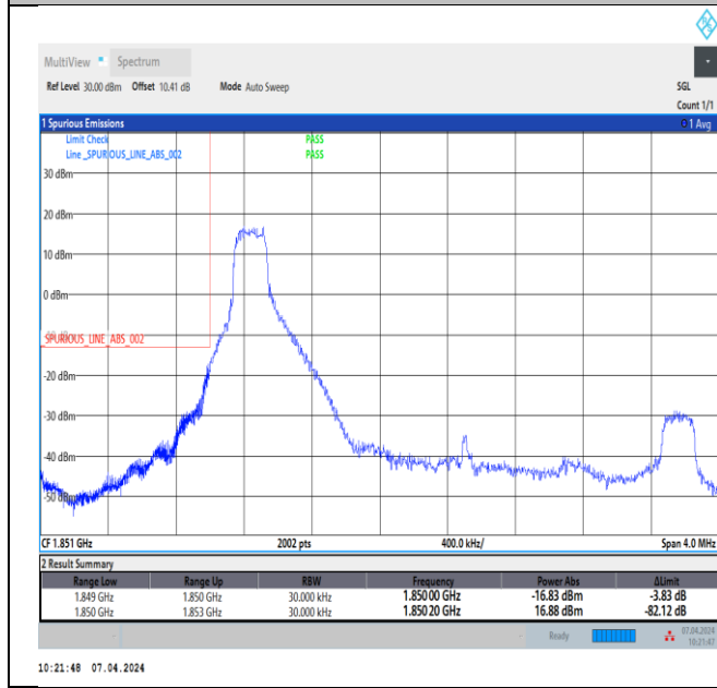
Band2_3MHz_QPSK_18615_1RB#0
