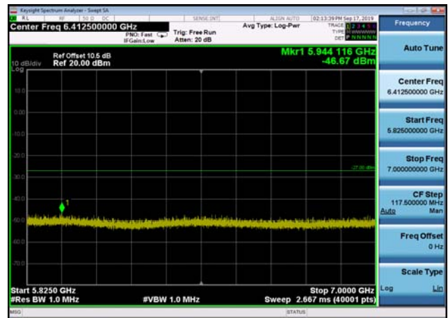
U-NII-1 ,Plot 3,5825MHz~7000MHz-802.1 1ac(80MHz),5210MHz,Ant2
