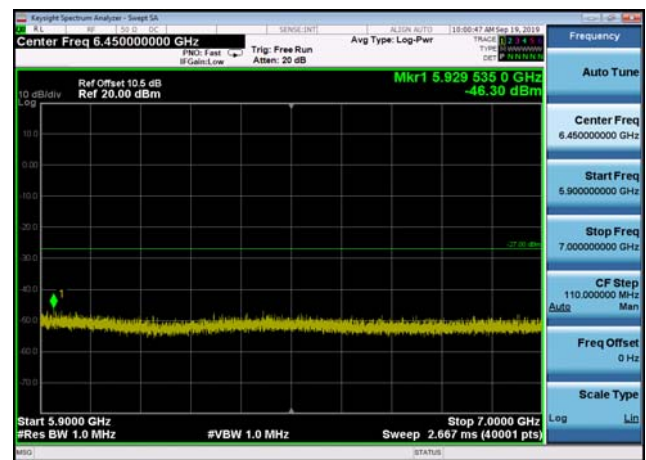
U-NII-3 ,Plot 3,5900MHz~7000MHz-802.1 1a(20MHz),5745MHz,Ant2
