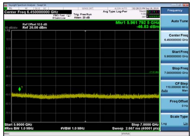
U-NII-3 ,Plot 3,5900MHz~7000MHz-802.1 1ac(20MHz),5825MHz,Ant2
