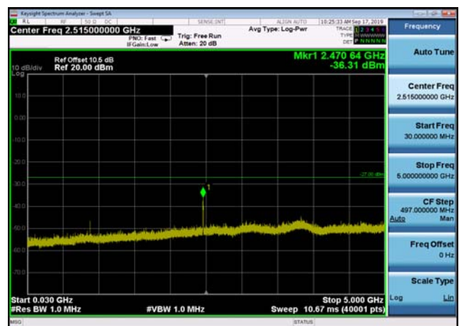
U-NII-1 ,Plot 2,30MHz~5000MHz-802.11a c(20MHz),5180MHz,Ant2
