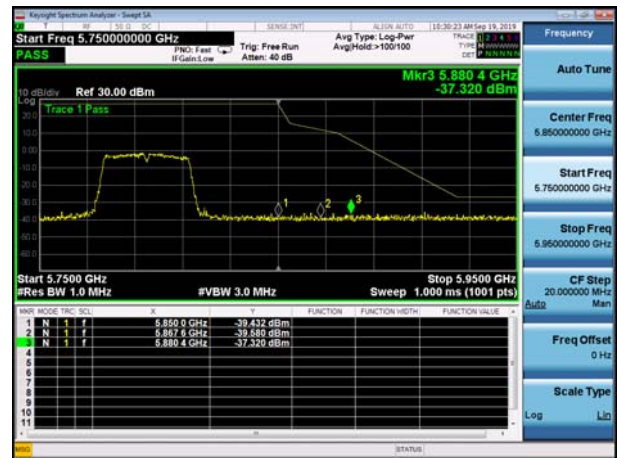
U-NII-3 Band Edge-802.11ac(40MHz) ,5795MHz, Ant2
