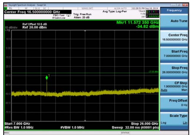
U-NII-3 ,Plot 4,7000MHz~26000MHz-802. 11ac(20MHz),5825MHz,Ant2
