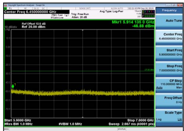
U-NII-3 ,Plot 3,5900MHz~7000MHz-802.1 1ac(40MHz),5755MHz,Ant2
