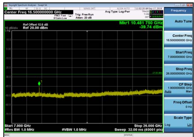
U-NII-1 ,Plot 4,7000MHz~26000MHz-802. 11ac(40MHz),5190MHz,Ant2
