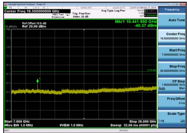
U-NII-1 ,Plot 4,7000MHz~26000MHz-802. 11ac(20MHz),5240MHz,Ant2
