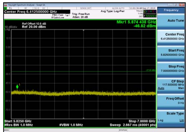
U-NII-1 ,Plot 3,5825MHz~7000MHz-802.1 1ac(40MHz),5190MHz,Ant2
