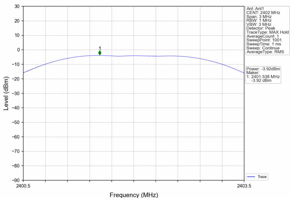
GFSK 2M LCH 240GFSK 2MHz Ant1 NTNV
