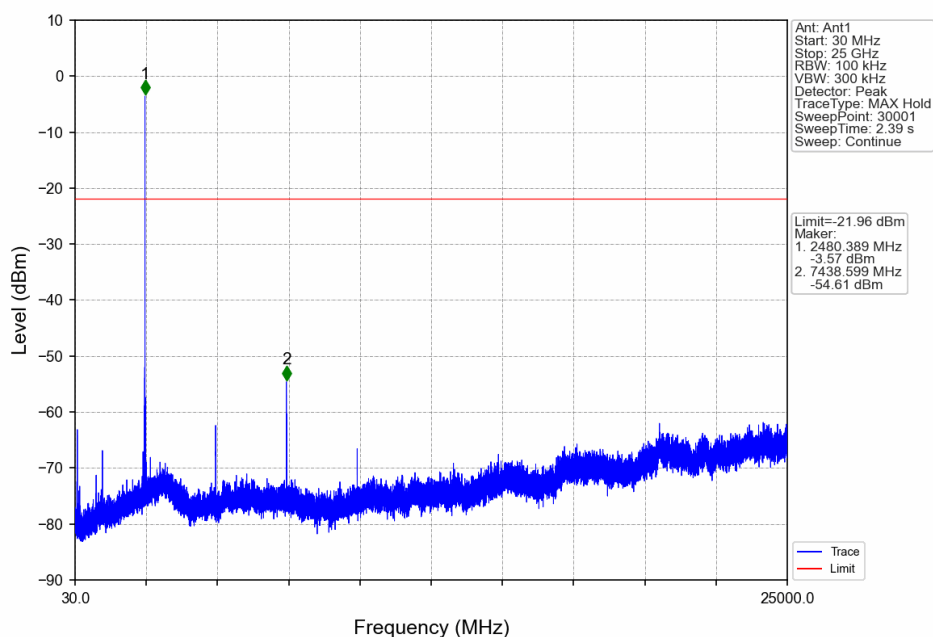
GFSK 2M HCH 2480MHz Ant1 NTN
