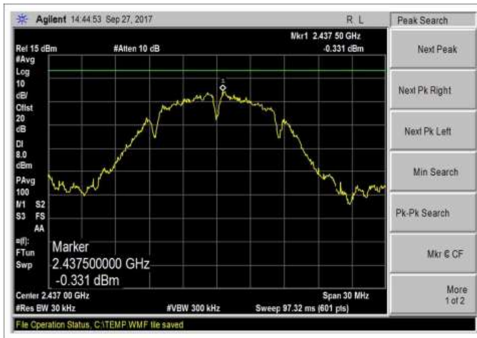
802.11b_PSD_Middle_CH6_2437MHz
