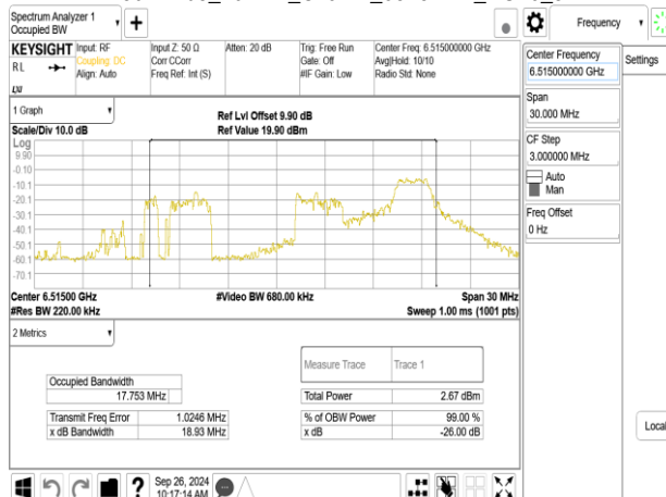
802.11be_20MHz_ChainB_6515MHz_RU26_8
