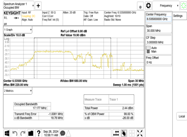
802.11be_20MHz_ChainB_6535MHz_RU26_0
