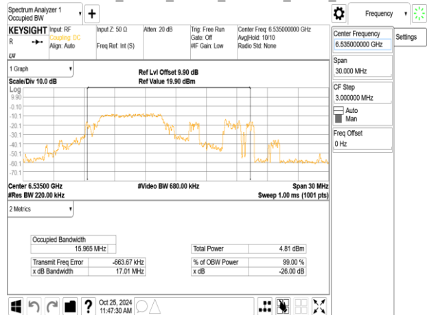
802.11be_20MHz_ChainB_6535MHz_RU106_53
