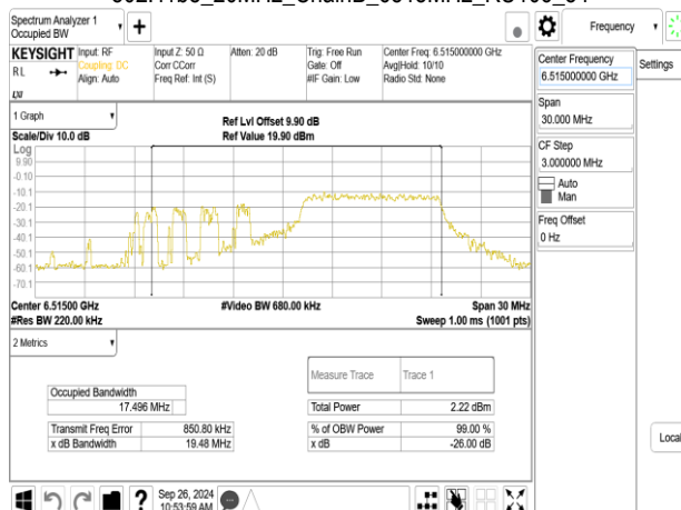
802.11be_20MHz_ChainB_6515MHz_RU26_8
