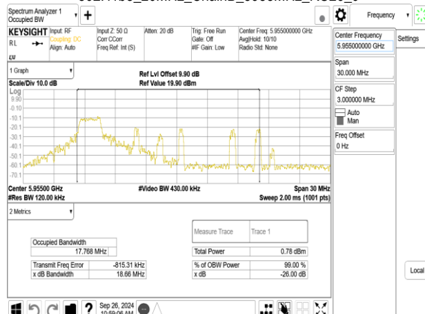
802.11be_20MHz_ChainB_5955MHz_RU52_37
