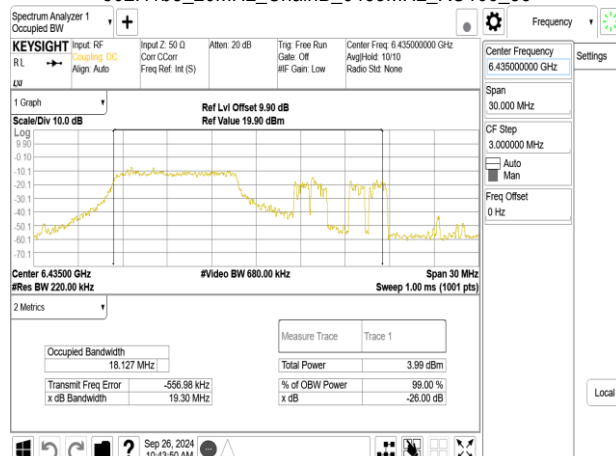
802.11be_20MHz_ChainB_6435MHz_RU26_0
