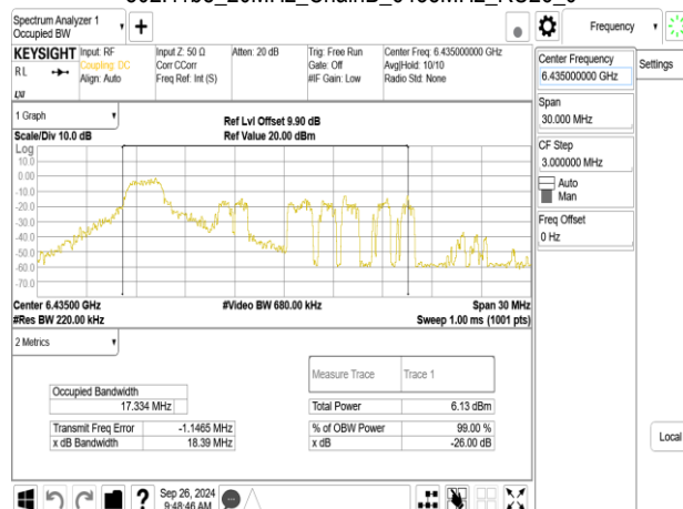
802.11be_20MHz_ChainB_6435MHz_RU52_37
