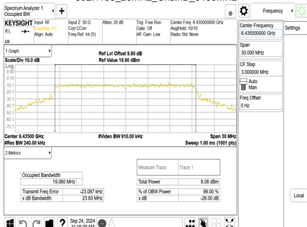
802.11be_20MHz_ChainB_6435MHz_106+26_MRU1
