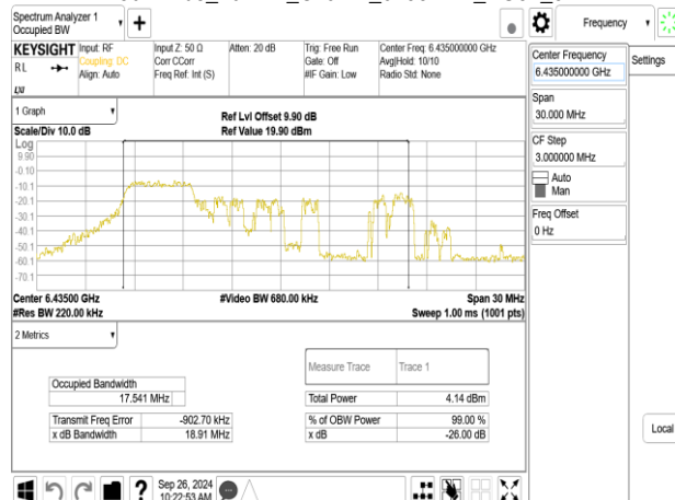
802.11be_20MHz_ChainB_6435MHz_RU52_37
