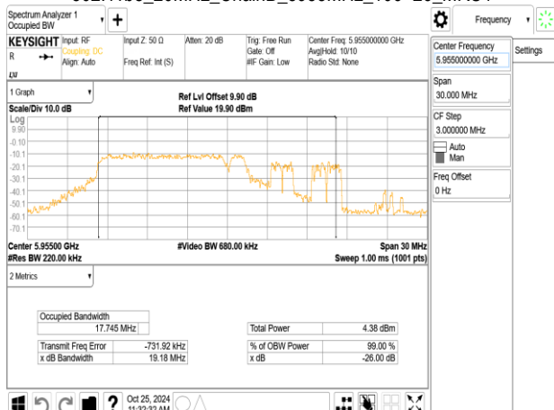
802.11be_20MHz_ChainB_5955MHz_52+26_MRU1
