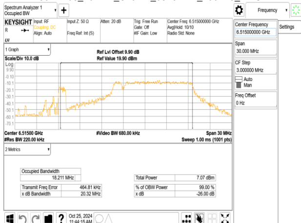
802.11be_20MHz_ChainB_6515MHz_106+26_MRUI2
