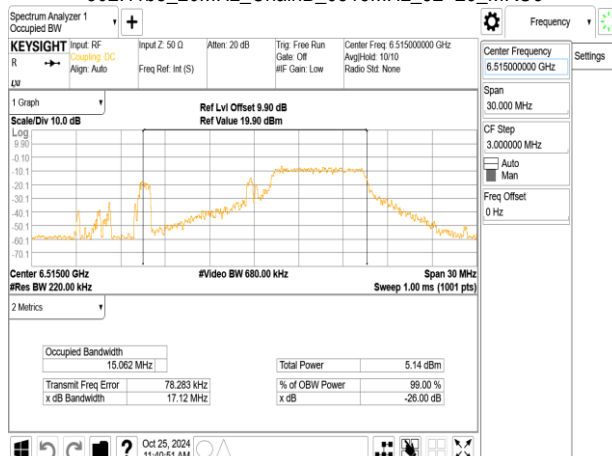
802.11be_20MHz_ChainB_6515MHz_RU106_54
