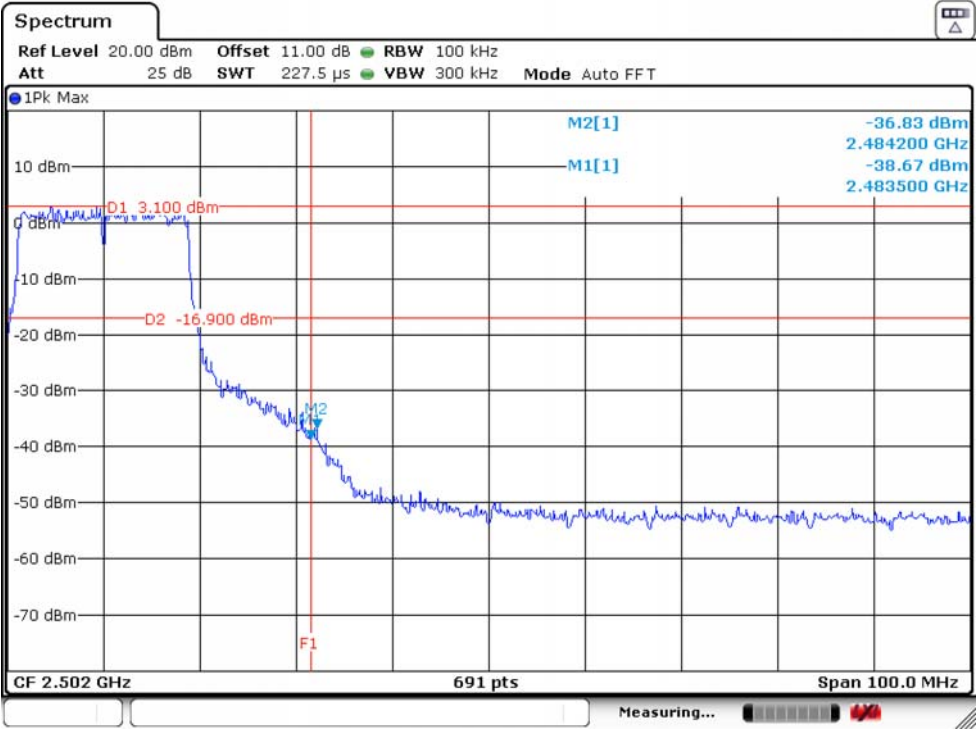
IEEE 802.11n HT20 2462MHz
