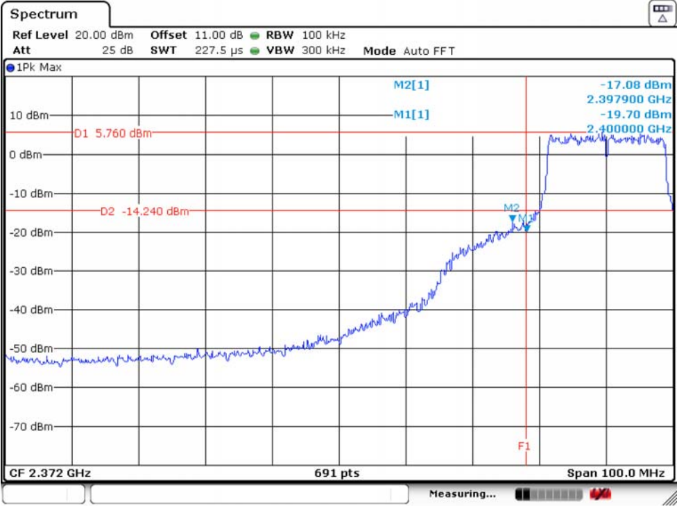
IEEE 802.11n HT20 2412MHz
