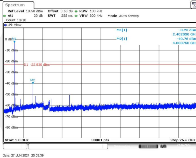
DH5_Ant1_2402_1000~26500
