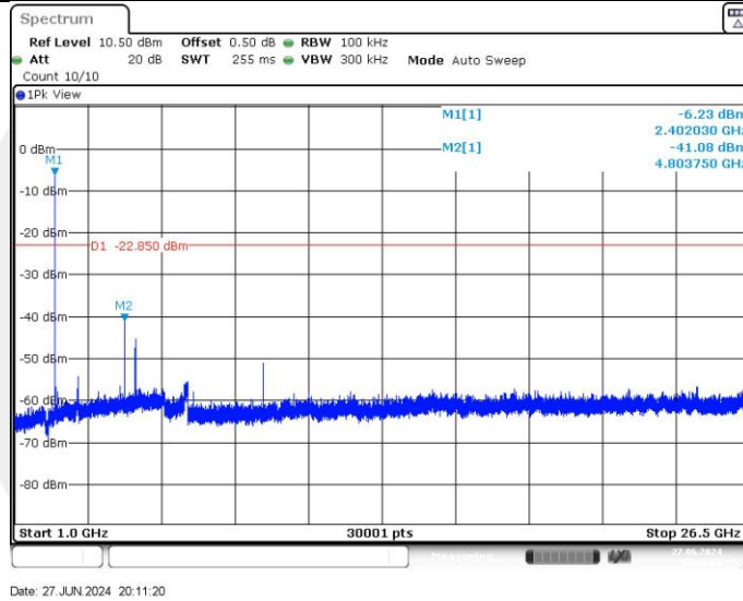
2DH5_Ant1_2402_1000~26500
