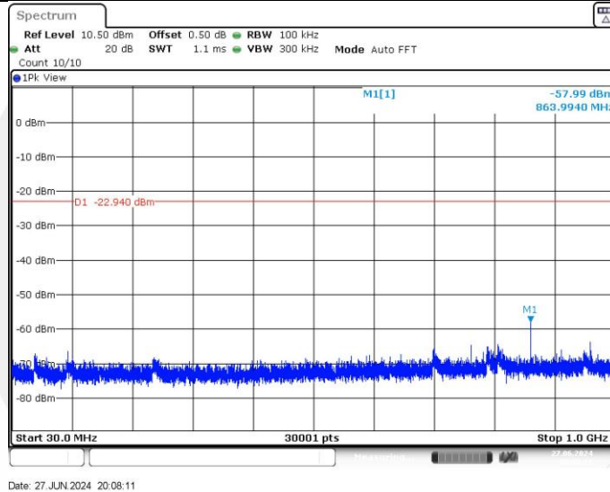
DH5_Ant1_2480_30~1000
