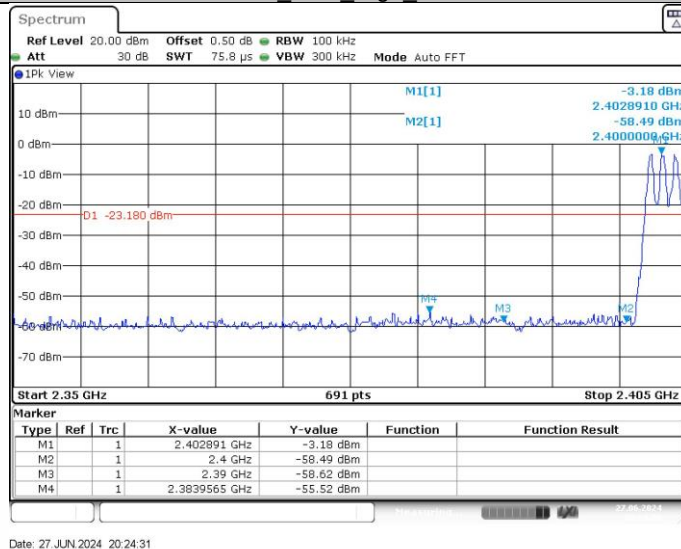
DH5_Ant1_Low_Hop_2402
