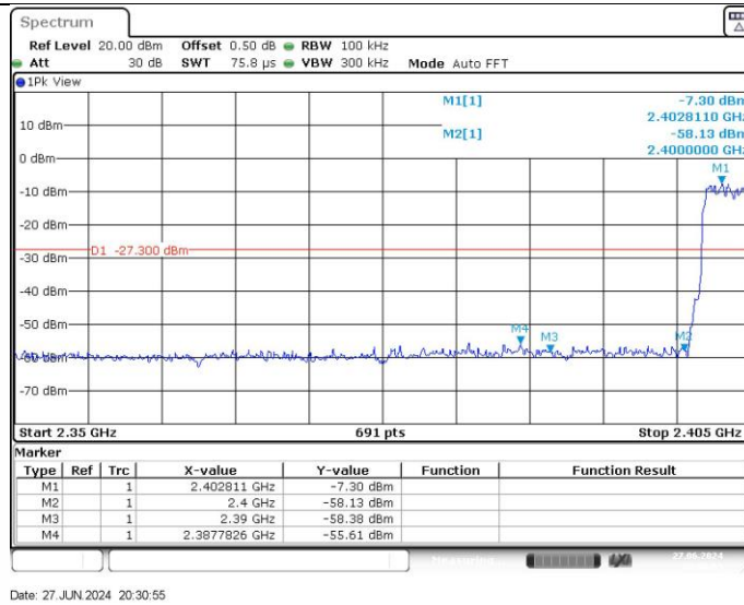
2DH5_Ant1_Low_Hop_2402
