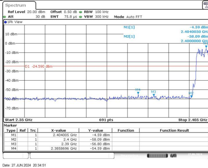
3DH5_Ant1_Low_Hop_2402
