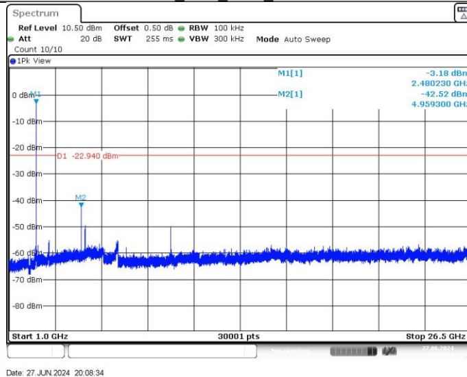
DH5_Ant1_2480_1000~26500
