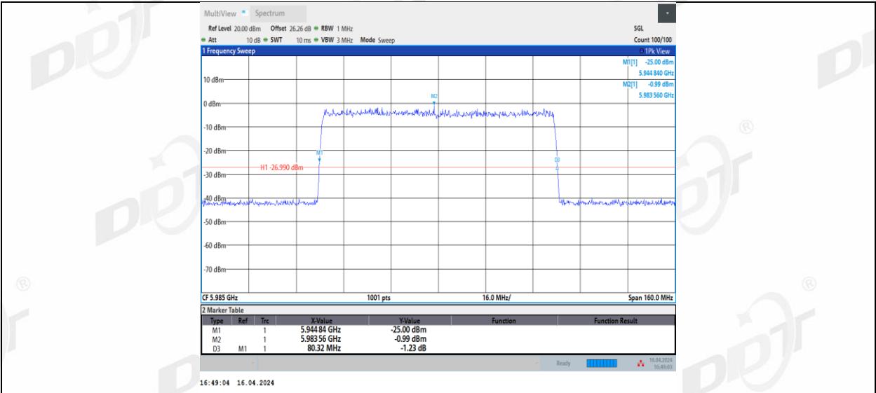
11AX80MIMO_Ant2_5985
