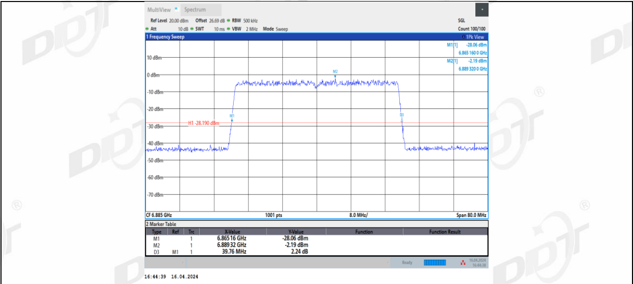
11AX40MIMO_Ant2_6885
