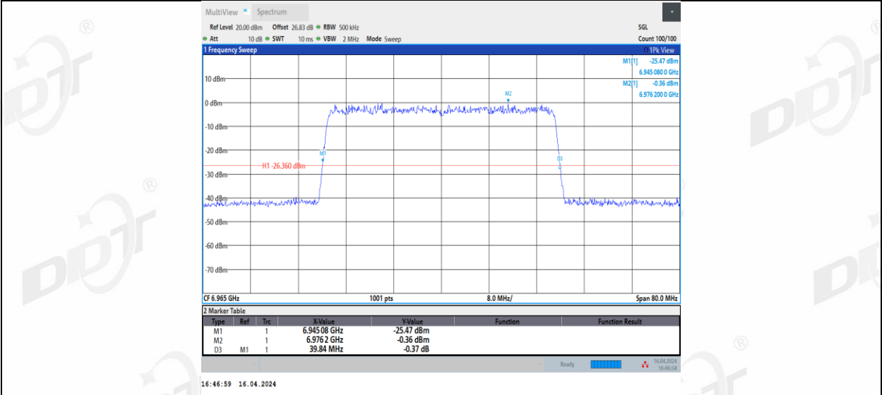
11AX40MIMO_Ant3_6965
