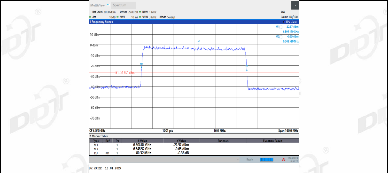
11AX80MIMO_Ant3_6545
