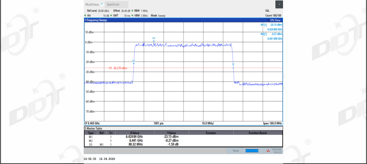
11AX80MIMO_Ant3_6465
