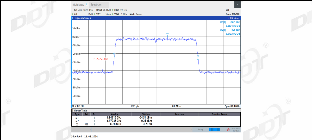
11AX40MIMO_Ant2_6965
