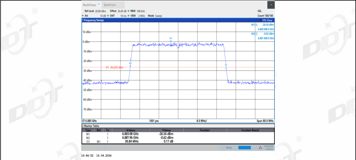
11AX40MIMO_Ant3_6885
