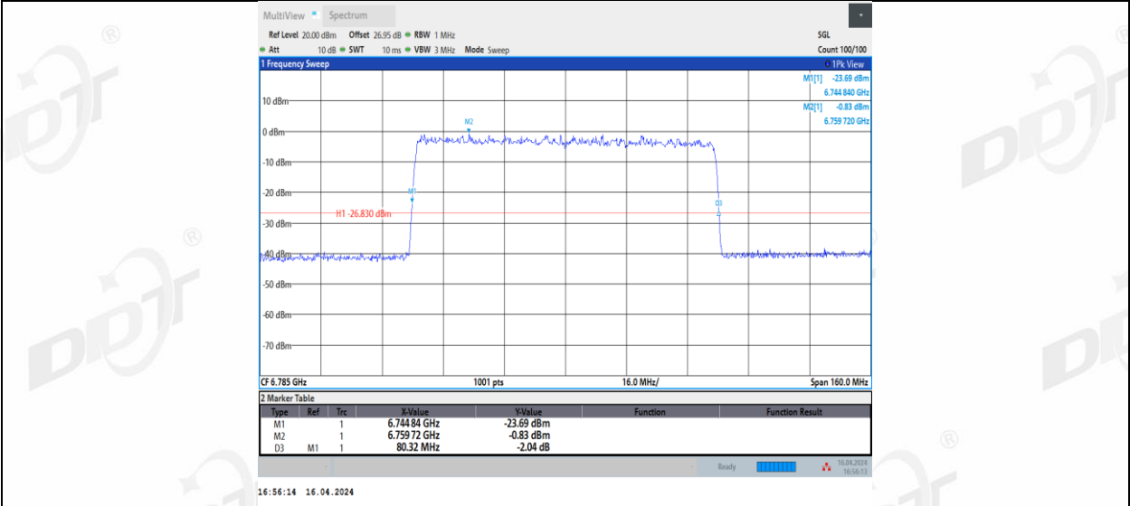
11AX80MIMO_Ant3_6785
