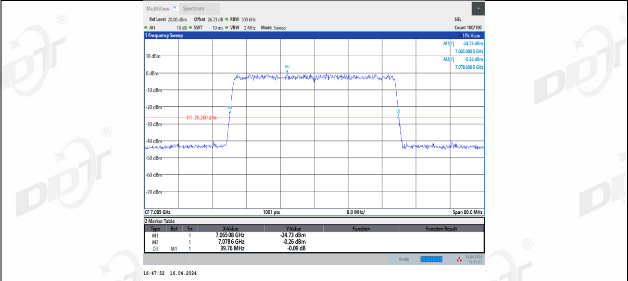
11AX40MIMO_Ant3_7085
