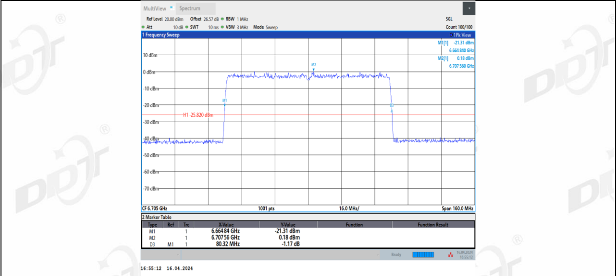
11AX80MIMO_Ant3_6705
