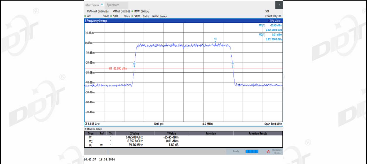
11AX40MIMO_Ant3_6845
