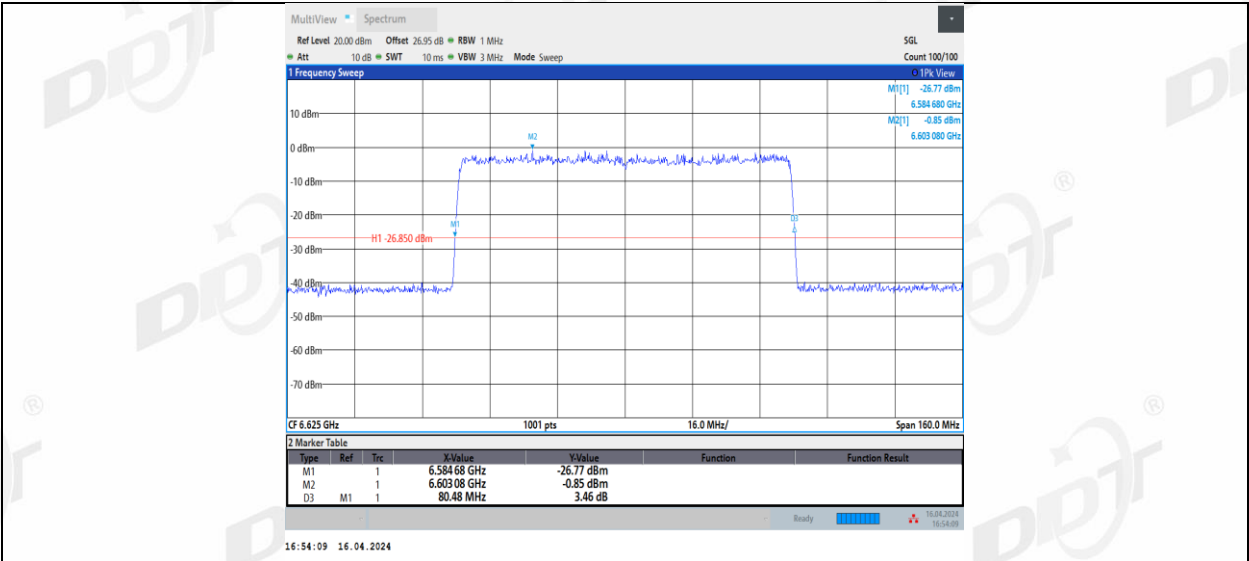
11AX80MIMO_Ant2_6625
