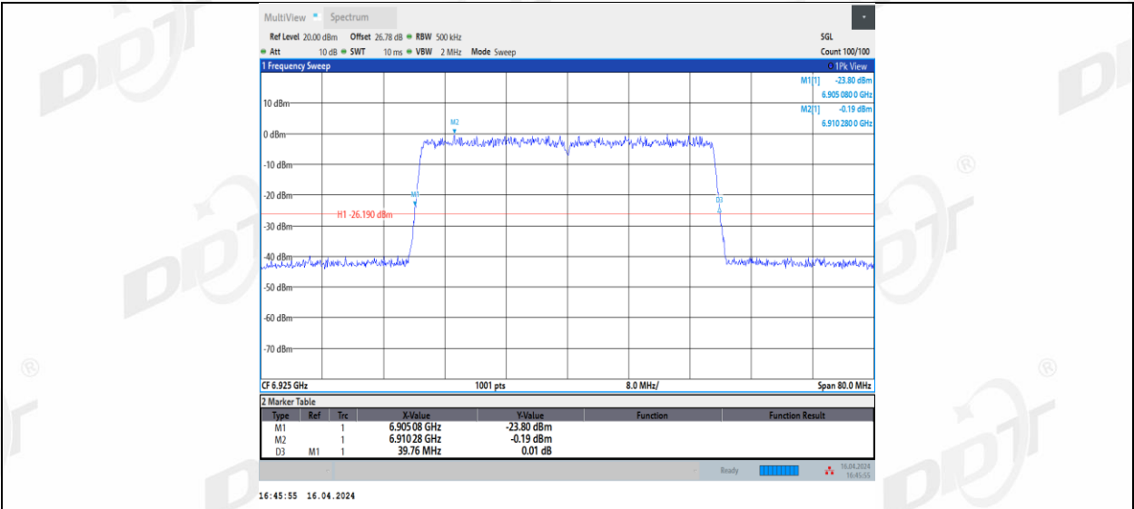
11AX40MIMO_Ant2_6925
