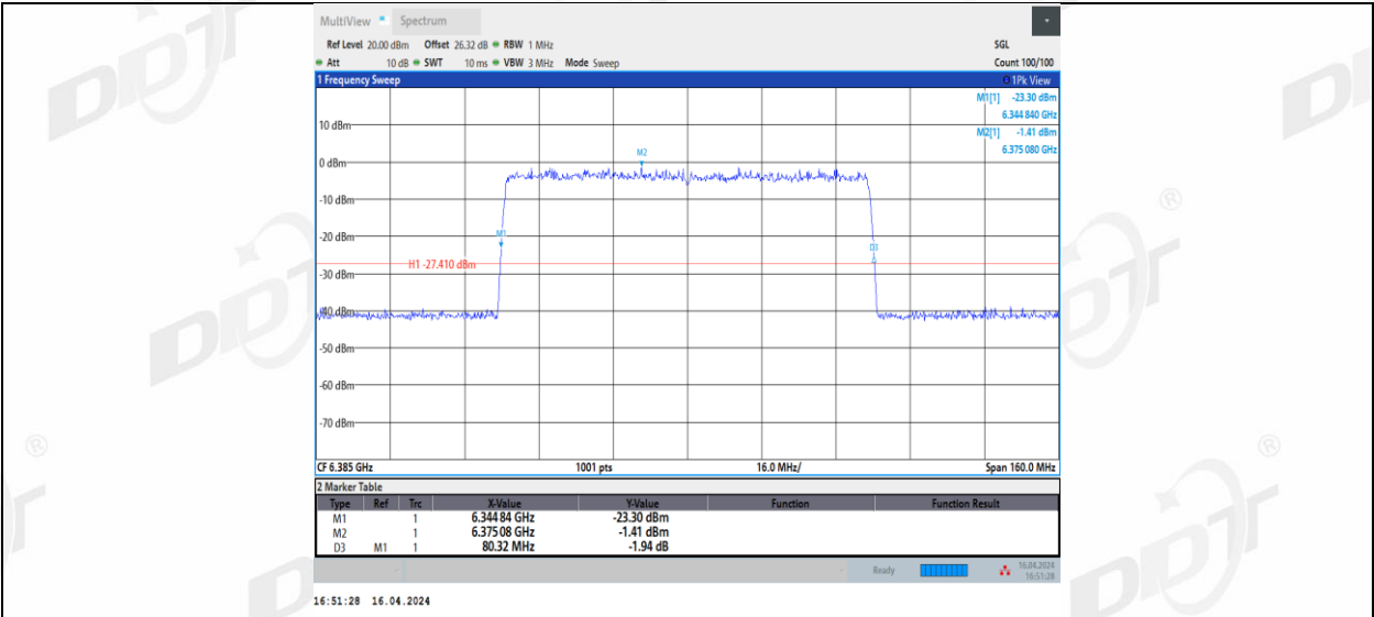
11AX80MIMO_Ant2_6385
