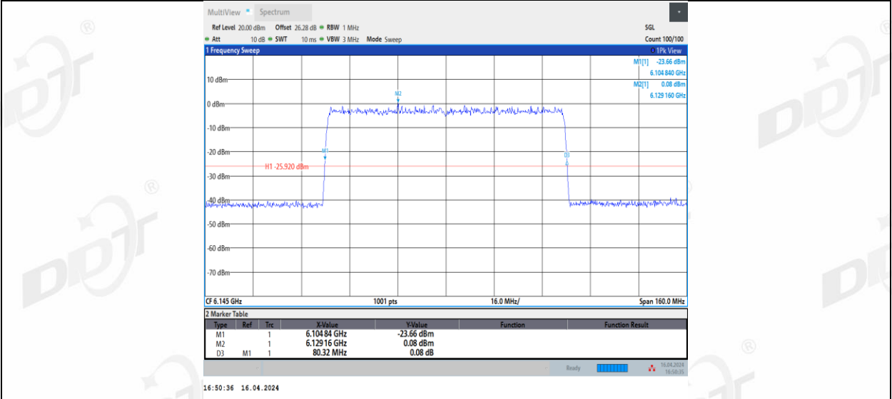
11AX80MIMO_Ant3_6145
