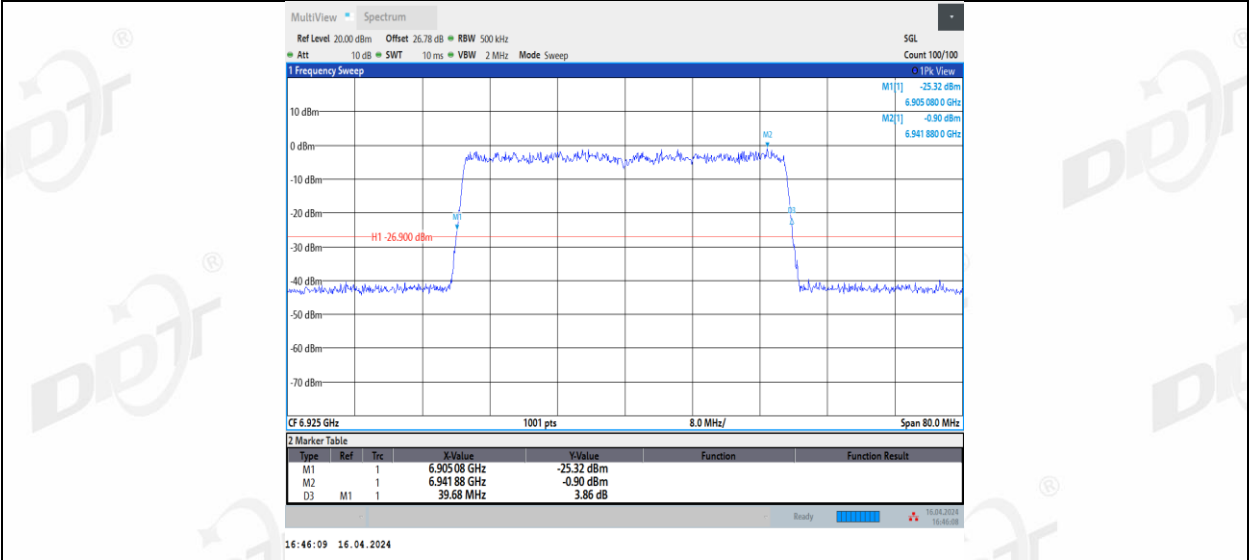
11AX40MIMO_Ant3_6925
