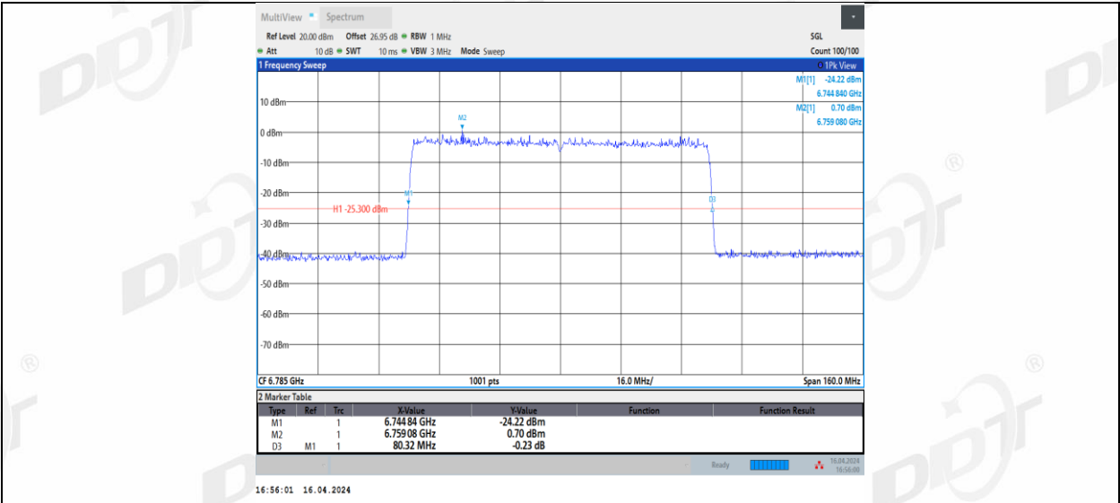
11AX80MIMO_Ant2_6785
