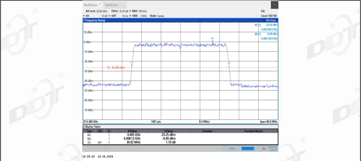
11AX40MIMO_Ant3_6485
