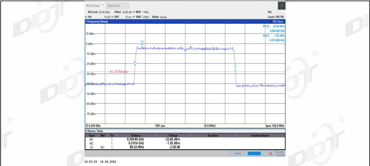
11AX80MIMO_Ant2_6545
