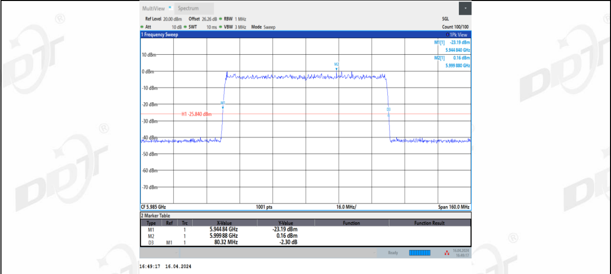
11AX80MIMO_Ant3_5985
