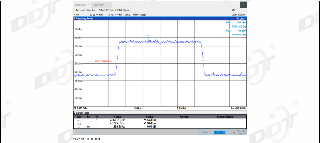
11AX40MIMO_Ant2_7085
