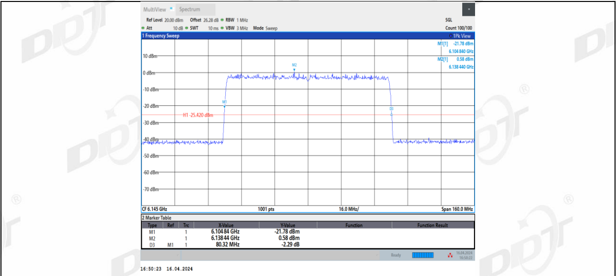
11AX80MIMO_Ant2_6145
