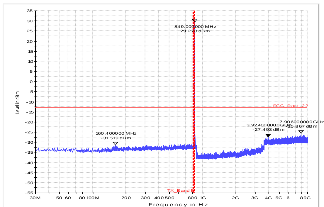
Fula2_FCC_22_GSM_Scan2_30MHz_9GHz
