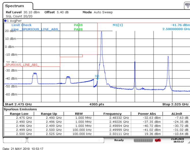
Band7_20MHz_16QAM_20850_100RB#0
