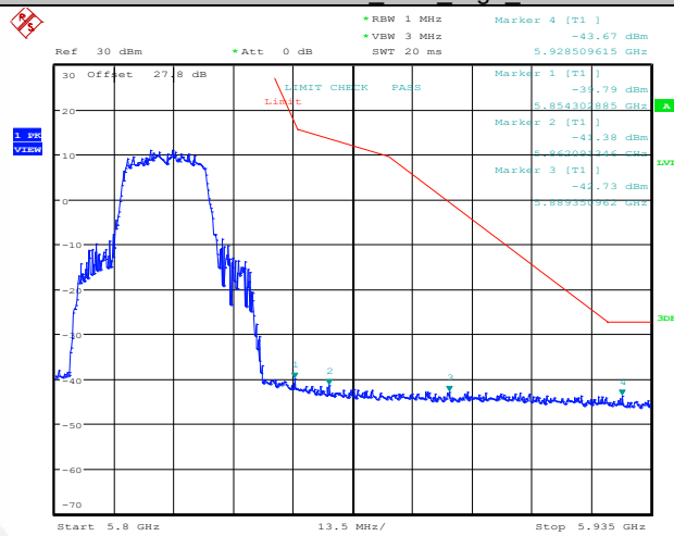
11AX20MIMO Ant1 High 5825
