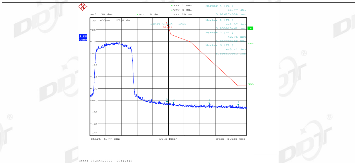
11AX40MIMO Ant1 High 5795
