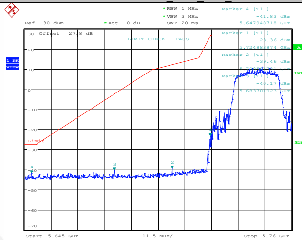
11AX20MIMO Ant1 Low 5745
