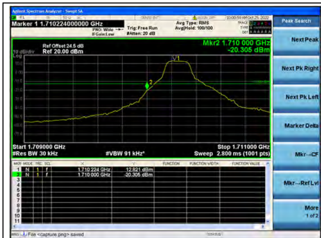
Band4 / 1.4MHz / Low CH / QPSK / 1 RB
