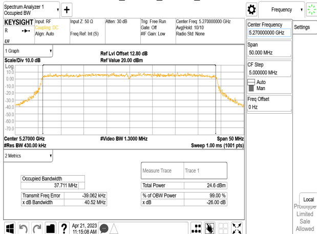
802.11ax_40MHz_Chain1_5270MHz
