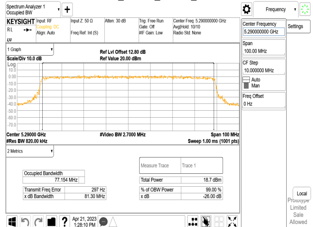
802.11ax_80MHz_Chain0_5290MHz
