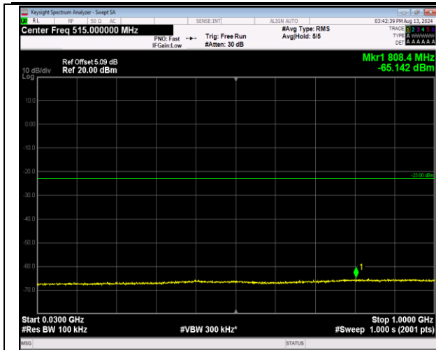
2-2-20MHz-20MHz-QPSK-QPSK-18700-18898-1RB#0-0 RB#0-30~1000MHz-PASS
