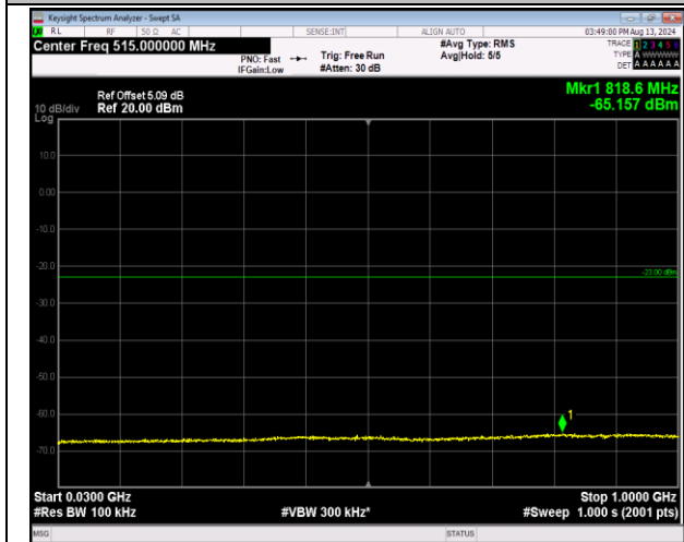
2-2-20MHz-20MHz-QPSK-QPSK-18801-18999-1RB#99-9 ORB#0-30~1000MHz-PASS
