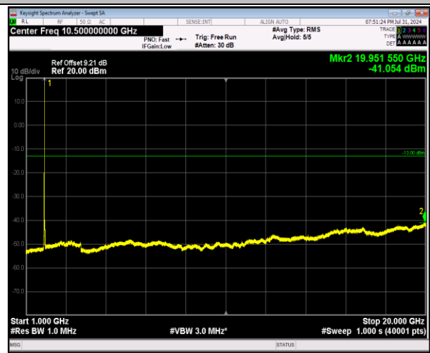
2-2-20MHz-20MHz-64QAM-64QAM-18801-18999-1RB#99- 0RB#0-1000~20000MHz-PASS
