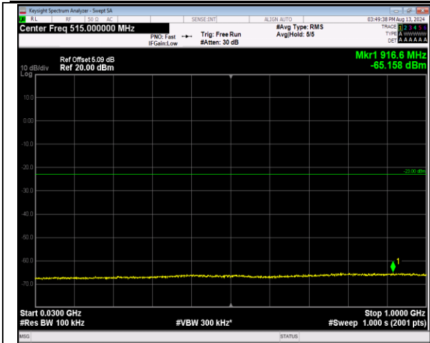
2-2-20MHz-20MHz-16QAM-16QAM-18801-18999-1RB#9 9-ORB#0-30~1000MHz-PASS
