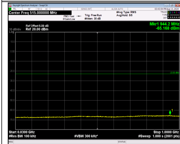
2-2-20MHz-20MHz-QPSK-QPSK-18700-18898-1RB#99-99 ORB#0-30~1000MHz-PASS
