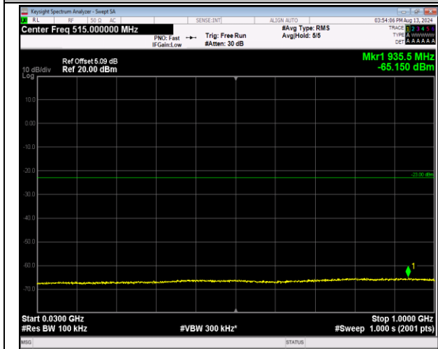
2-2-20MHz-20MHz-QPSK-QPSK-18902-19100-1RB#99-99 ORB#0-30~1000MHz-PASS
