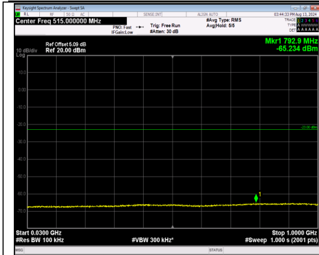
2-2-20MHz-20MHz-16QAM-16QAM-18700-18898-1RB#9 9-ORB#0-30~1000MHz-PASS
