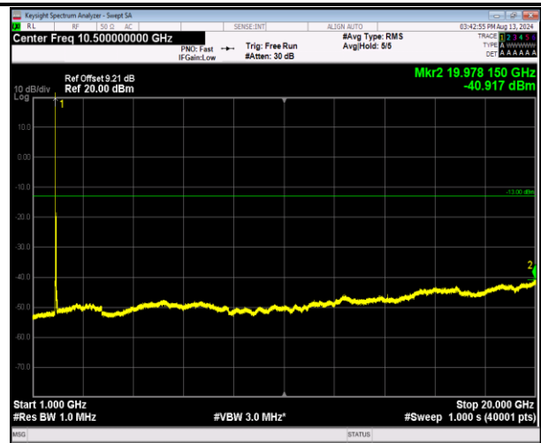
2-2-20MHz-20MHz-QPSK-QPSK-18700-18898-1RB#0-0RB #0-1000~20000MHz-PASS
