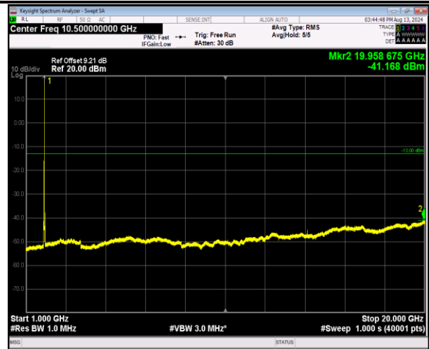
2-2-20MHz-20MHz-16QAM-16QAM-18700-18898-1RB#99- ORB#0-1000~20000MHz-PASS
