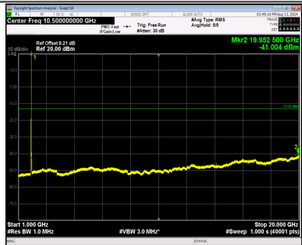
2-2-20MHz-20MHz-QPSK-QPSK-18801-18999-1RB#99-0R B#0-1000~20000MHz-PASS
