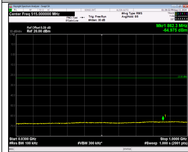
2-2-5MHz-20MHz-QPSK-QPSK-18983-19100-1RB#0-1R B#99-30~1000MHz-PASS
