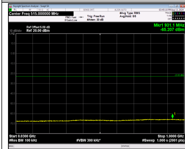
2-2-20MHz-20MHz-QPSK-QPSK-18700-18898-1RB#0-1 RB#99-30~1000MHz-PASS
