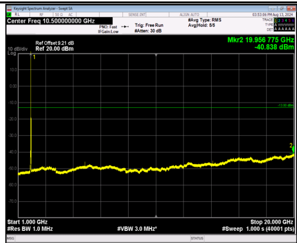
2-2-20MHz-20MHz-QPSK-QPSK-18902-19100-1RB#0-0RB #0-1000~20000MHz-PASS
