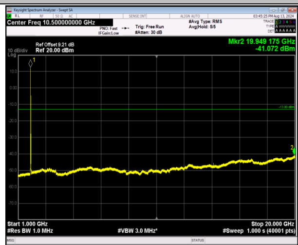
2-2-20MHz-20MHz-QPSK-QPSK-18700-18898-1RB#0-1RB #99-1000~20000MHz-PASS
