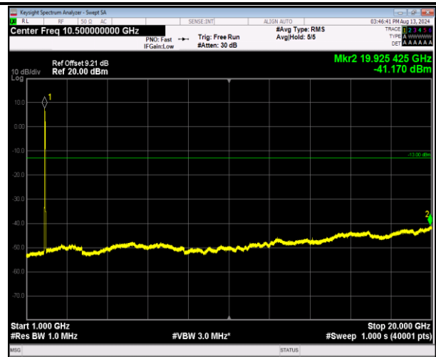
2-2-20MHz-20MHz-QPSK-QPSK-18700-18898-100RB#0-1 00RB#0-1000~20000MHz-PASS
