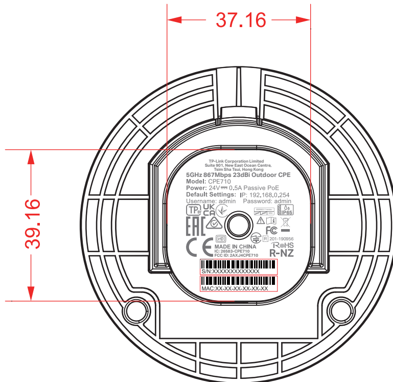
尺寸圖
