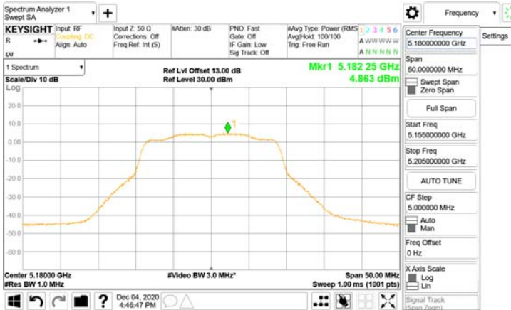
802.11n_20MHz_Chain1_5180MHz-5180
