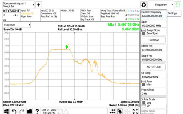
802.11ax_20MHz_Chian0_5500MHz-106-53
