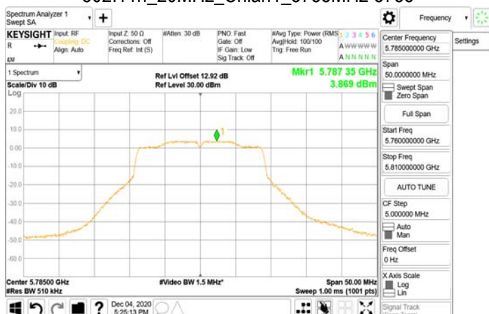
802.11n_20MHz_Chian1_5785MHz-5785
