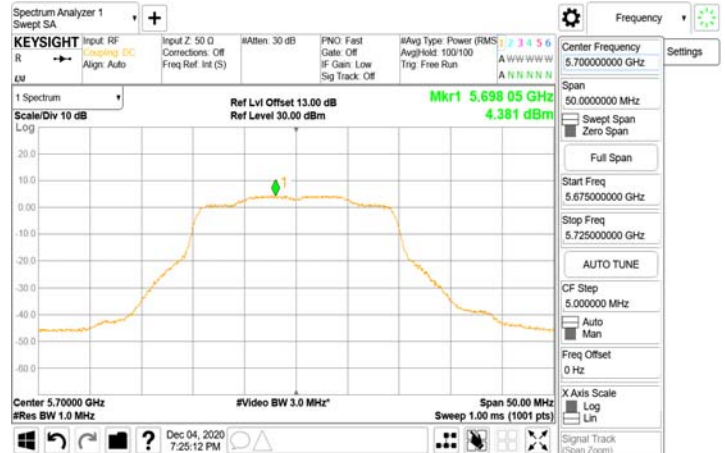
802.11ax_20MHz_Chian0_5700MHz-106-54
