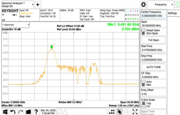
802.11ax_20MHz_Chain0_5500MHz-52-37
