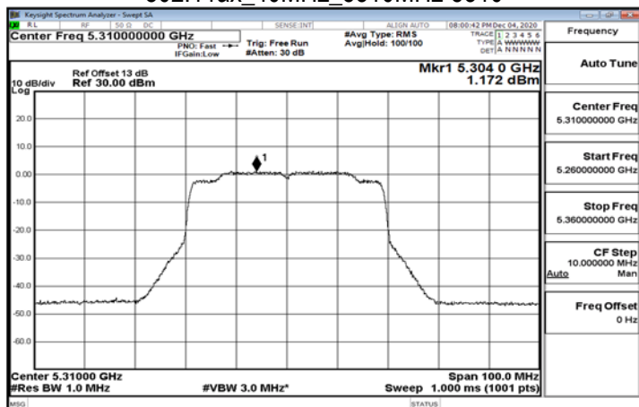
802.11ax_40MHz_5310MHz-242-62
