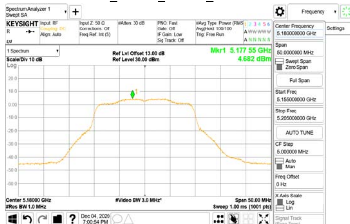
802.11ax_20MHz_Chain0_5180MHz-106-53
