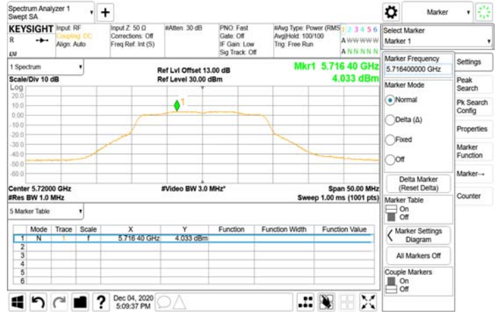
802.11n_20MHz_Chain0_5720MHz_UNII 3
