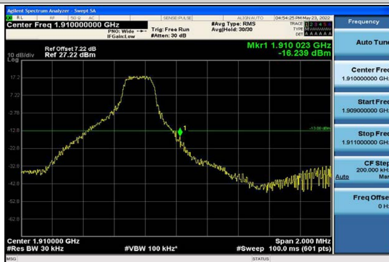
Band2-3MHz-QPSK-19185-1RB#14
