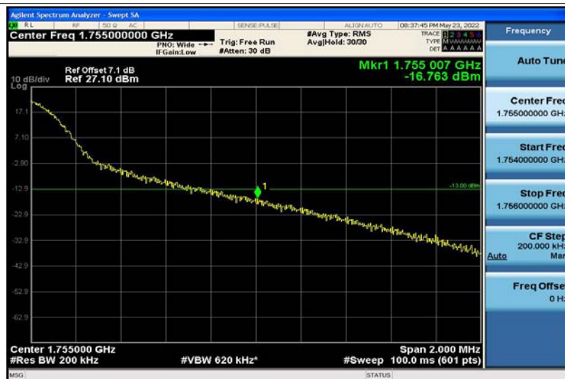
Band4-20MHz-QPSK-20300-1RB#99
