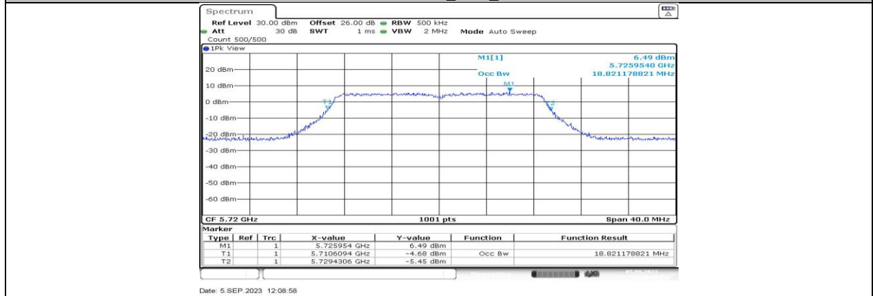
11AC20MIMO_Ant2_5720
