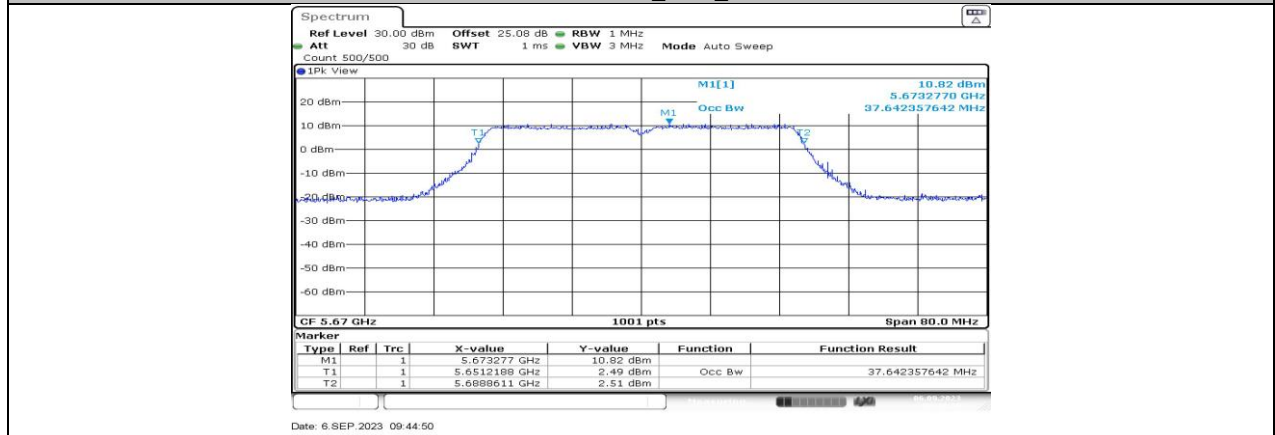
11AC40MIMO_Ant3_5670
