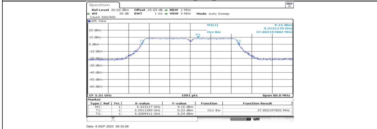
11AC40MIMO_Ant1_5310
