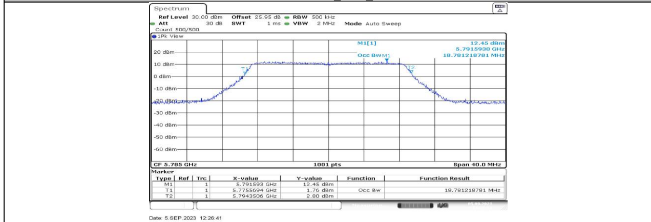
11AC20MIMO_Ant1_5785
