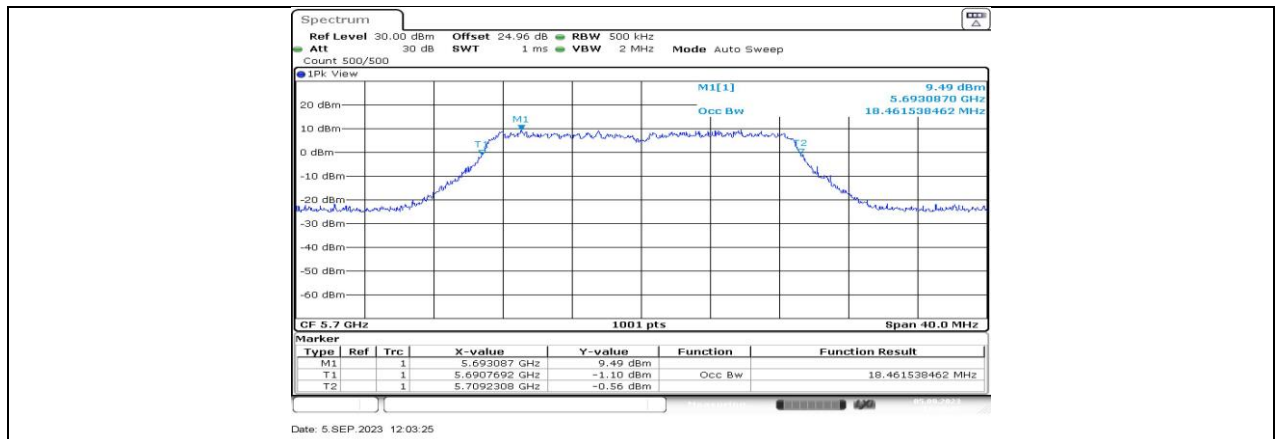
11AC20MIMO_Ant4_5700
