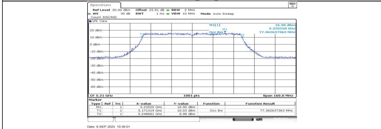
11AC80MIMO_Ant2_5210
