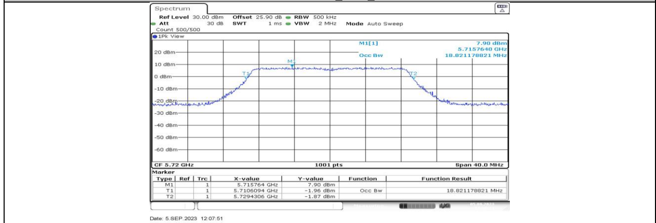
11AC20MIMO_Ant1_5720
