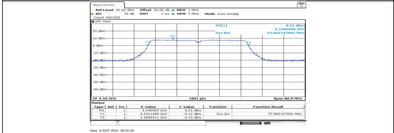
11AC40MIMO_Ant1_5550
