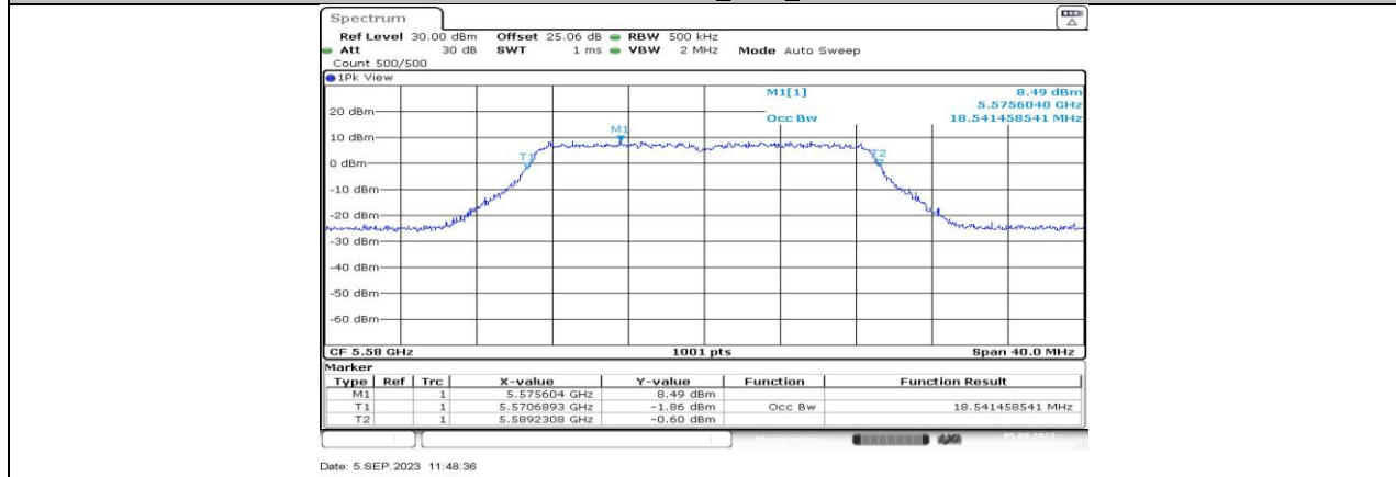
11AC20MIMO_Ant3_5580
