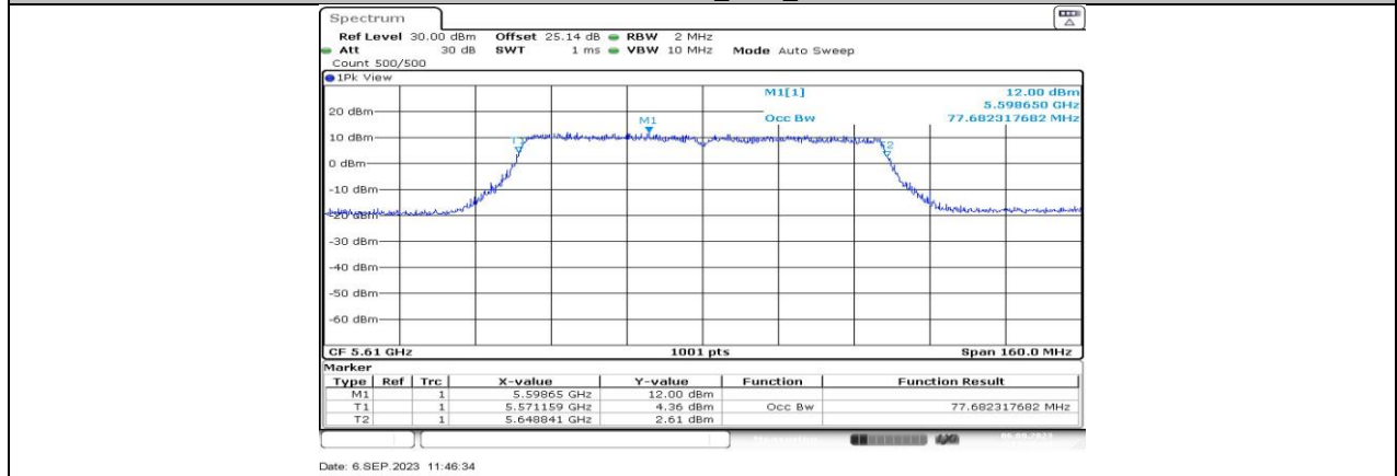
11AC80MIMO_Ant3_5610
