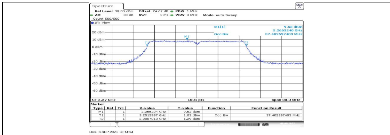
11AC40MIMO_Ant4_5270
