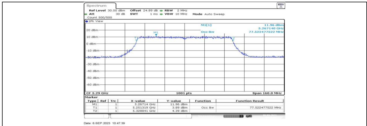
11AC80MIMO_Ant3_5290
