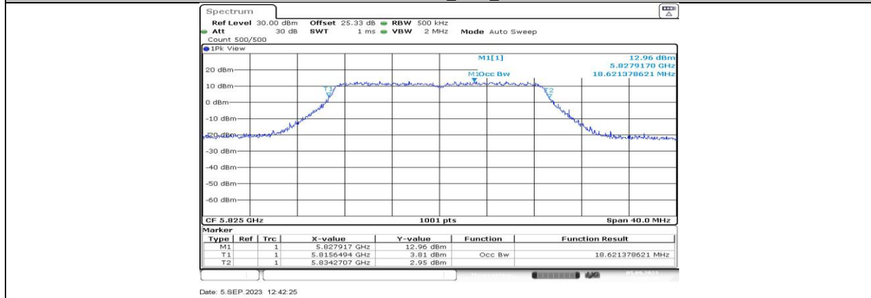
11AC20MIMO_Ant3_5825
