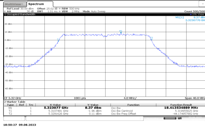
11AC20MIMO_Ant3_5320
