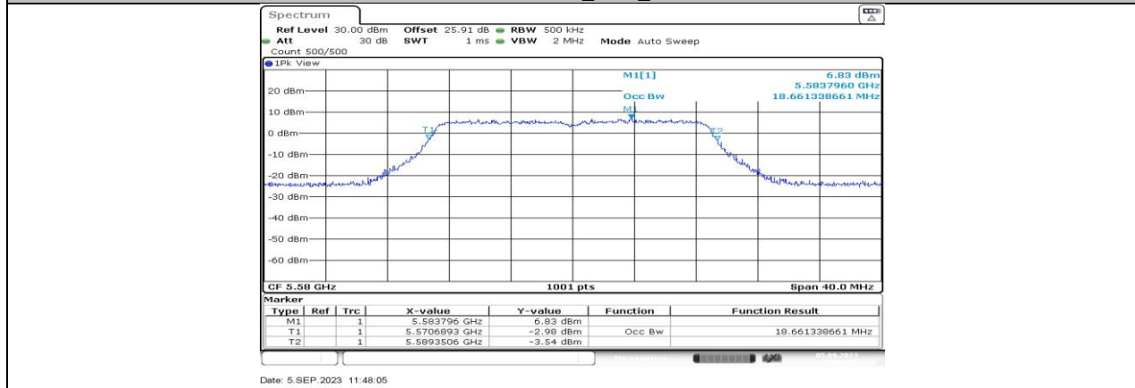
11AC20MIMO_Ant2_5580
