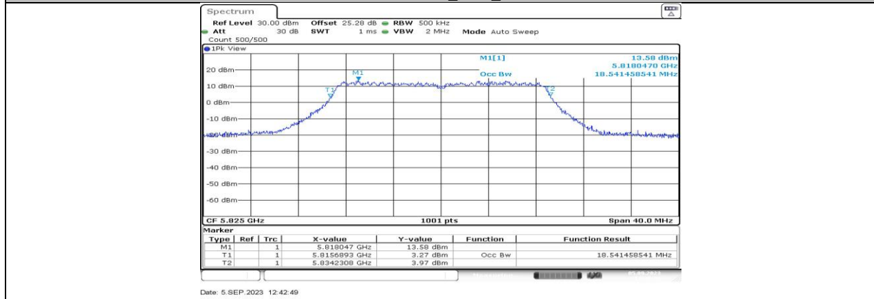
11AC20MIMO_Ant4_5825
