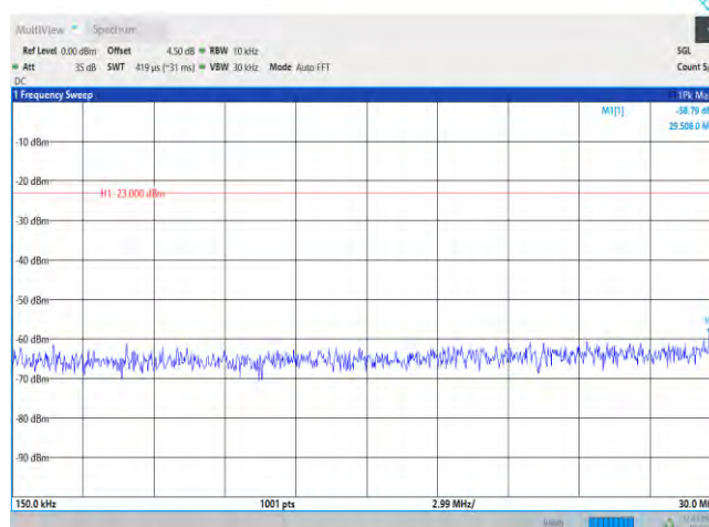
Band4-20MHz-QPSK-20050-1RB#0-Range2:0.15~30MHz
