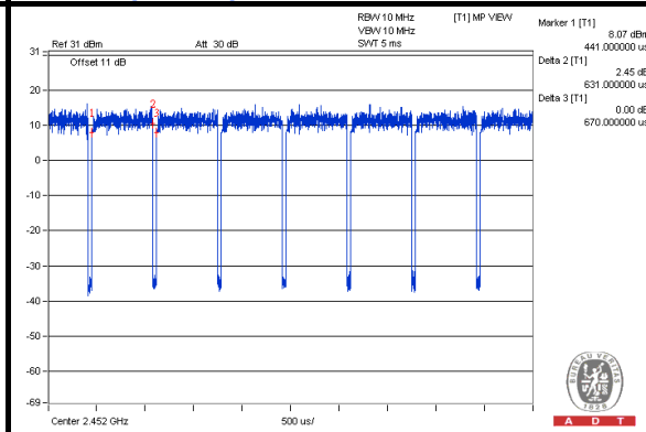
802.11n (40MHz)
