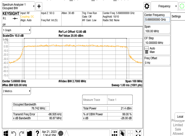
802.11ax_80MHz_Chain1_5690MHz
