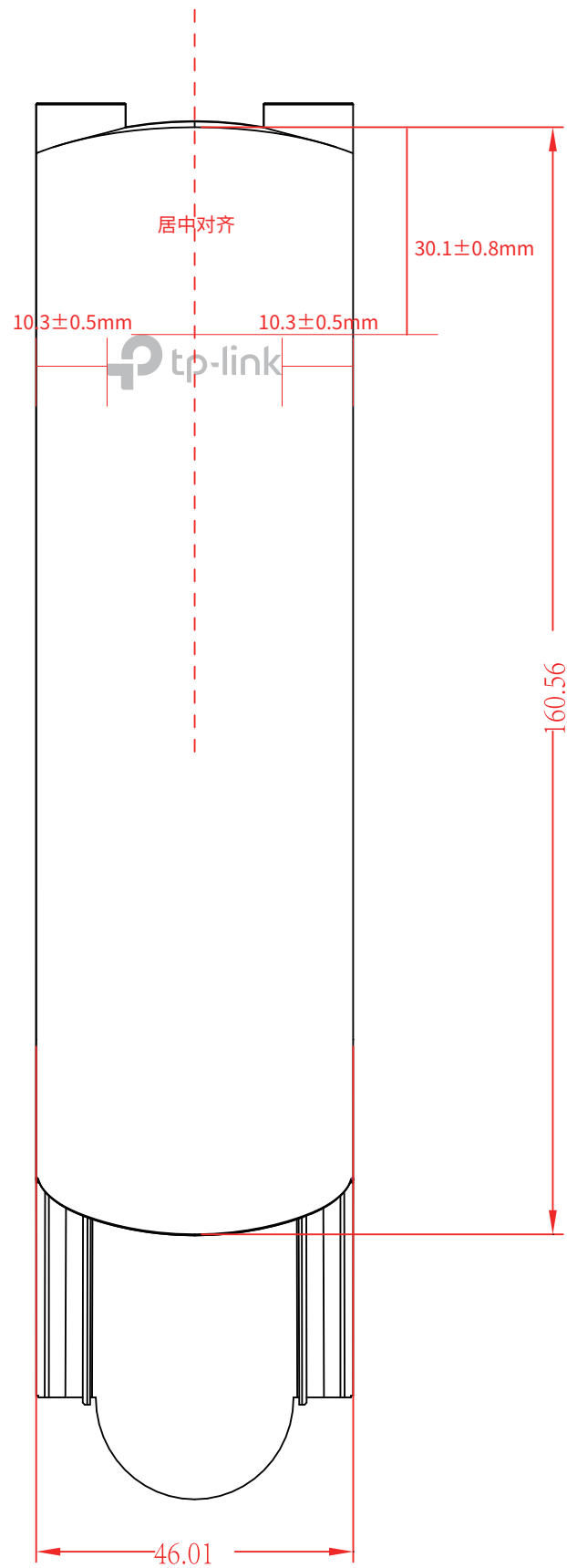
尺寸图
