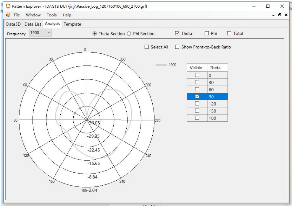
LTE B2 G1900 W1900 Theta=90deg
