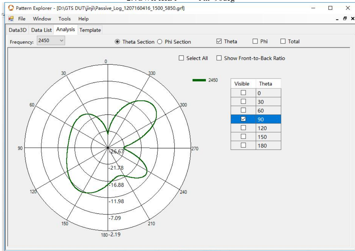
2.4GWIFI&BT Theta=90d
