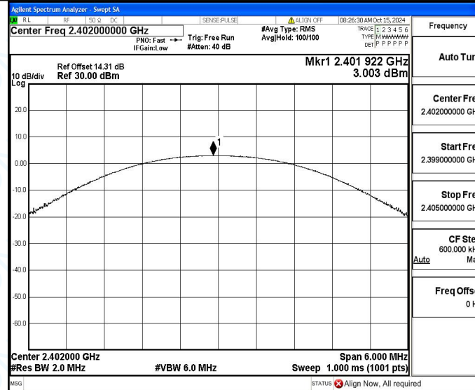
DH5 Ant1 2402
