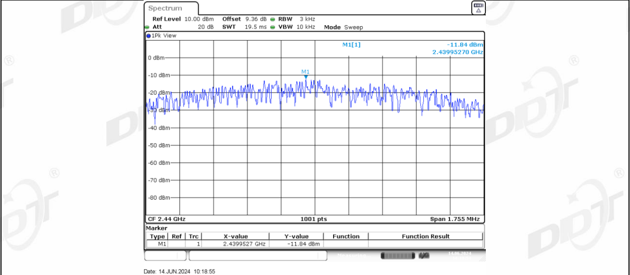
BLE_2M_Right side_2440
