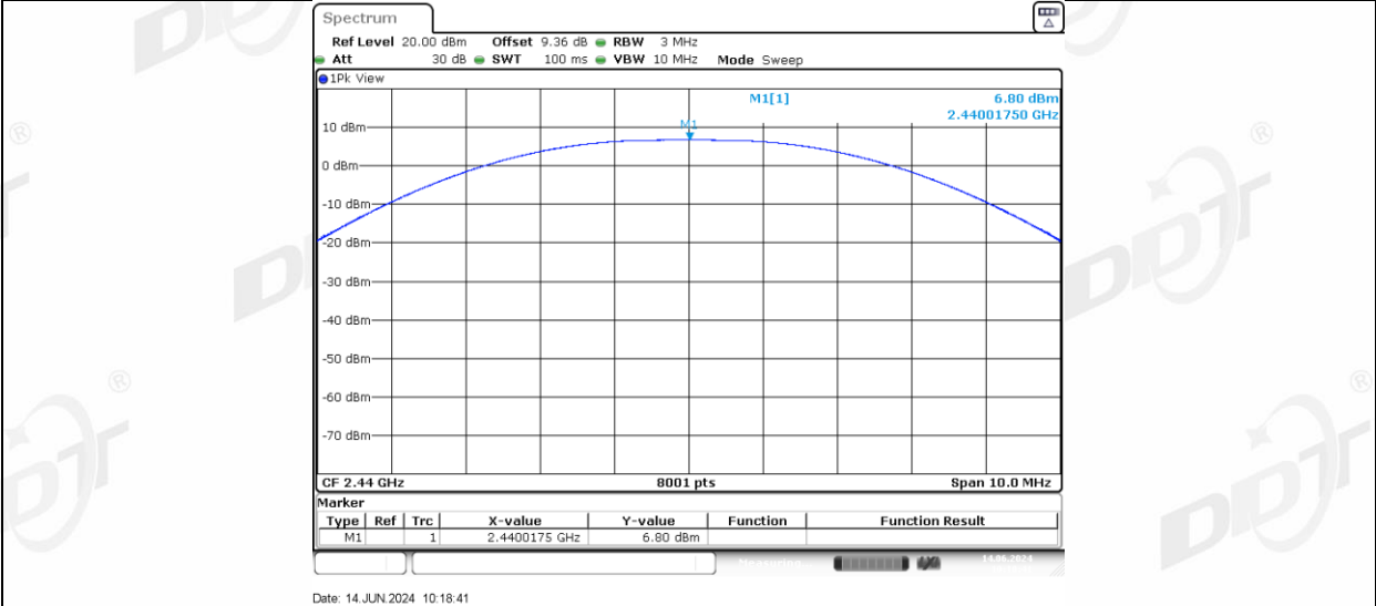
BLE_2M_Right side_2440
