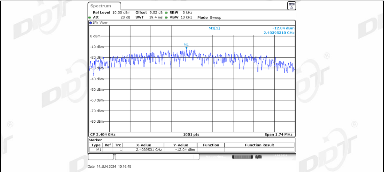
BLE_2M_Right side_2404
