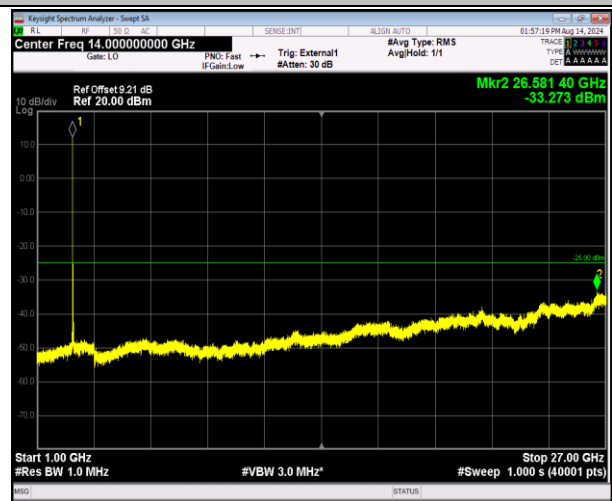
41-41-20MHz-5MHz-QPSK-QPSK-41090-41207-1RB#0-01RB#24-1000~27000MHz-PASS
