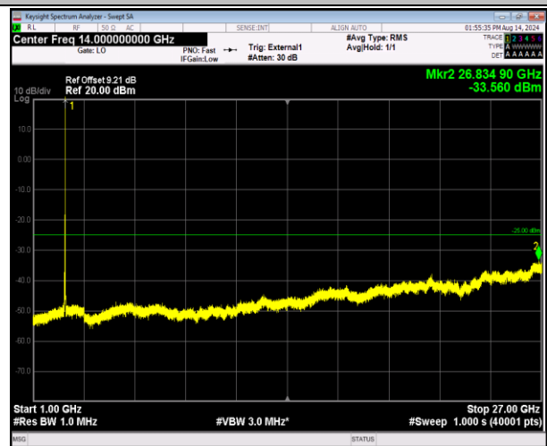
41-41-20MHz-5MHz-QPSK-QPSK-41090-41207-1RB#99-0RB#0-1000~27000MHz-PASS
