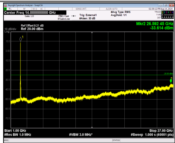
41-41-20MHz-20MHz-QPSK-QPSK-40340-40538-1RB#0-1 RB#99-1000~27000MHz-PASS
