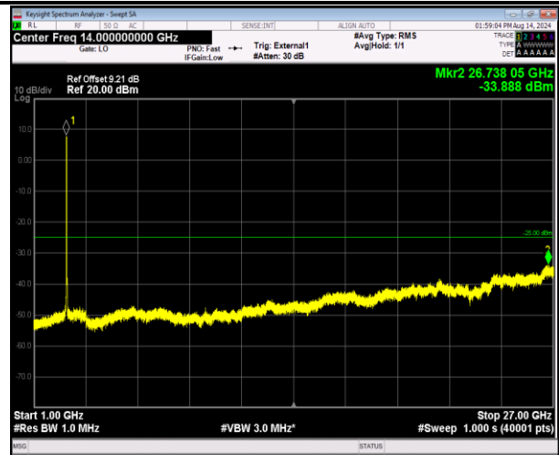
41-41-20MHz-5MHz-QPSK-QPSK-41090-41207-100RB#0- 25RB#0-1000~27000MHz-PASS
