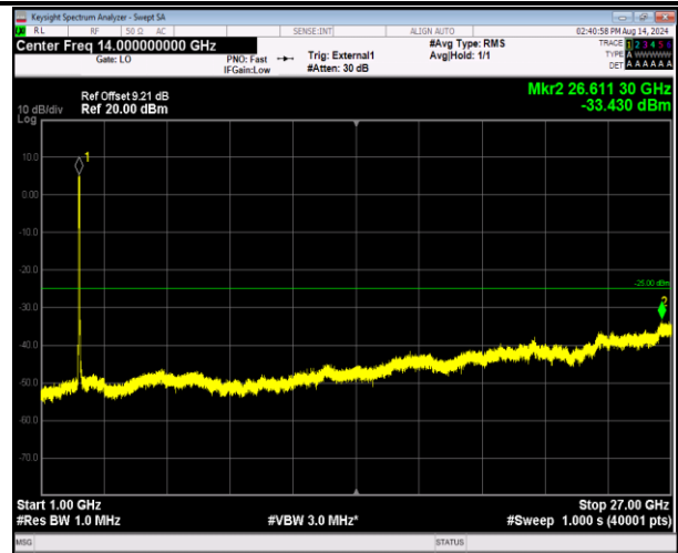
41-41-20MHz-20MHz-QPSK-QPSK-40340-40538-100RB#0 -100RB#0-1000~27000MHz-PASS
