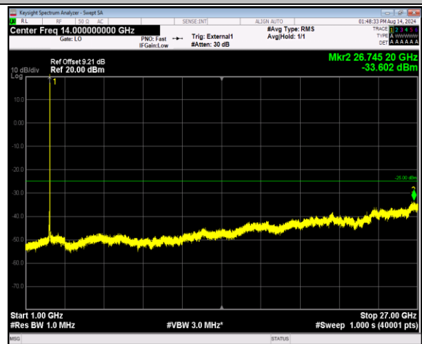
41-41-20MHz-5MHz-QPSK-QPSK-40715-40832-1RB#99-0RB#0-1000~27000MHz-PASS
