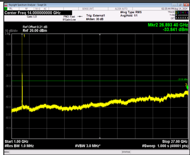
41-41-20MHz-20MHz-QPSK-QPSK-40340-40538-1RB#0-0 RB#0-1000~27000MHz-PASS
