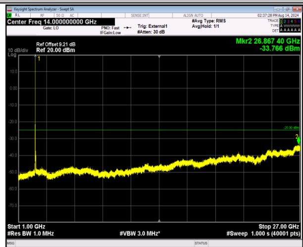
41-41-20MHz-20MHz-QPSK-QPSK-40340-40538-1RB#99- ORB#0-1000~27000MHz-PASS
