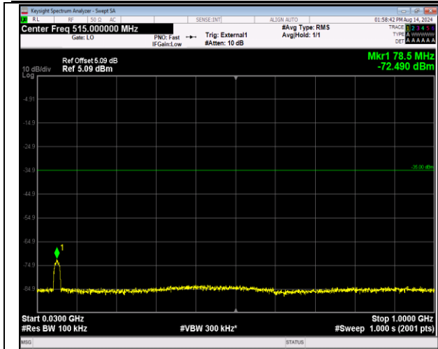
41-41-20MHz-5MHz-QPSK-QPSK-41090-41207-100RB# 0-25RB#0-30~1000MHz-PASS
