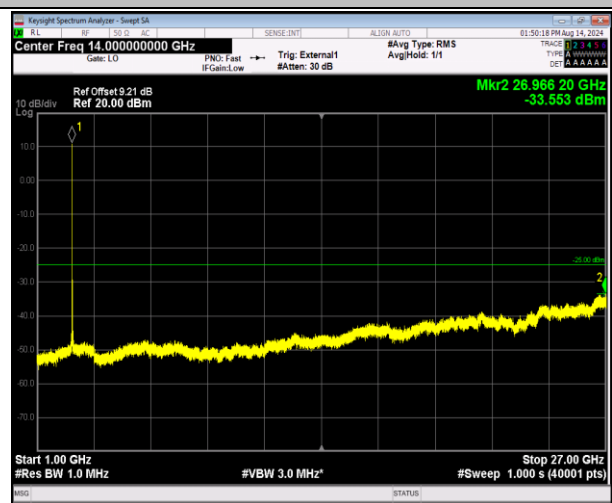
41-41-20MHz-5MHz-QPSK-QPSK-40715-40832-1RB#0-01RB#24-1000~27000MHz-PASS
