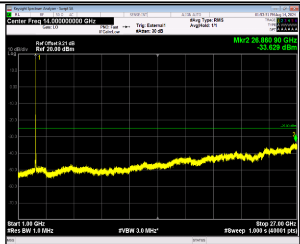
41-41-20MHz-5MHz-QPSK-QPSK-41090-41207-1RB#0-0RB#0-1000~27000MHz-PASS
