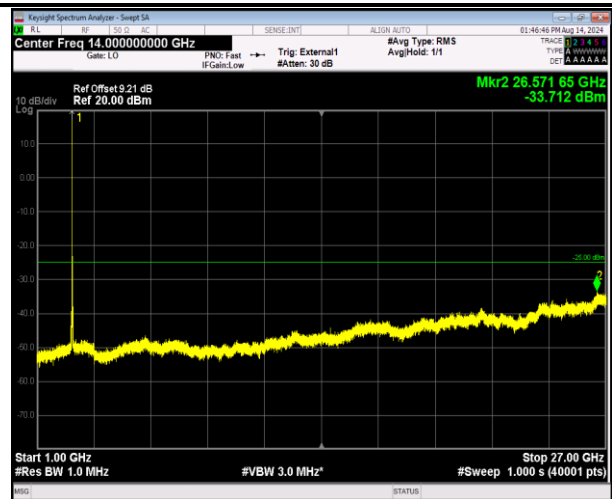
41-41-20MHz-5MHz-QPSK-QPSK-40715-40832-1RB#0-0RB#0-1000~27000MHz-PASS
