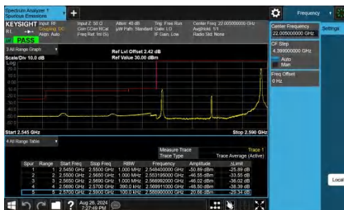
Band38-20MHz-QPSK-37850-1RB#99-PASS
