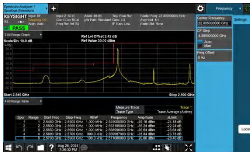
Band38-20MHz-QPSK-37850-1RB#0-PASS
