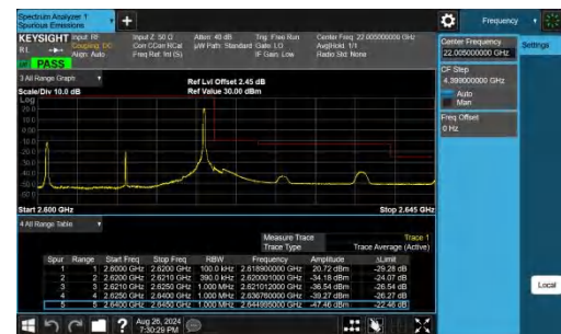
Band38-20MHz-QPSK-38150-1RB#99-PASS
