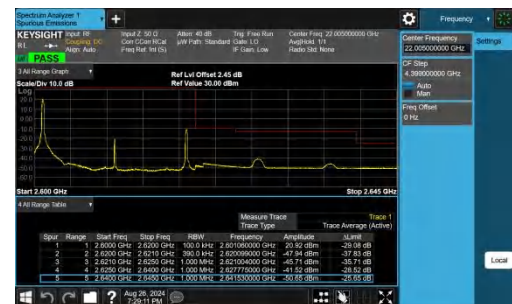
Band38-20MHz-QPSK-38150-1RB#0-PASS
