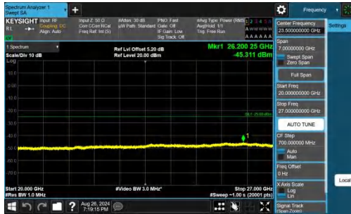
Band38-15MHz-QPSK-37825-1RB#0-20000~27000-PASS
