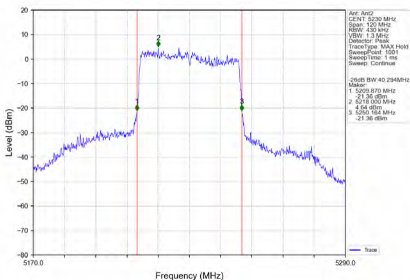
802.11ax(HE40) HCH 5230MHz RU484 Left Ant2 NTNv
