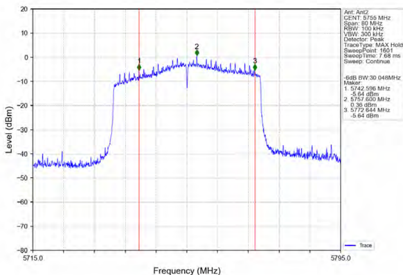
802.11ax(HE40) LCH 5755MHz RU484 Left Ant2 NTN
