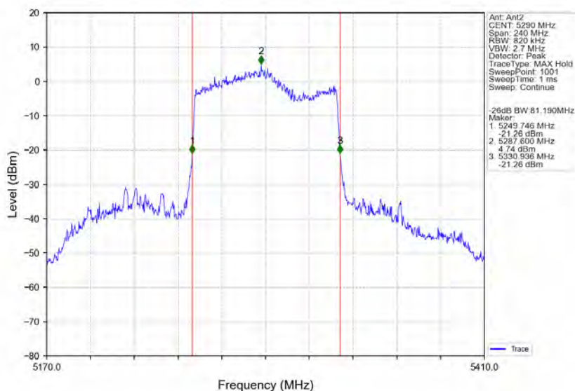
802.11ax(HE80) MCH 5290MHz RU996 Left Ant2 NTN
