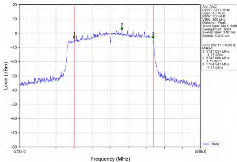
802.11ax(HE20) LCH 5745MHz RU242 Left Ant2 NTN
