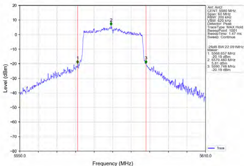
802.11ax(HE20) MCH 5580MHz RU242 Left Ant2 NTN
