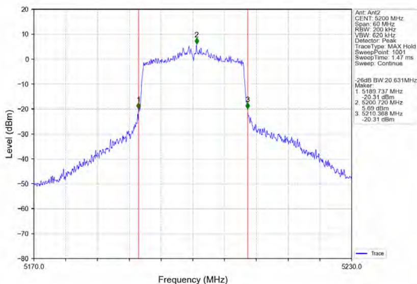
802.11ax(HE20) MCH 5200MHz RU242 Left Ant2 NTN
