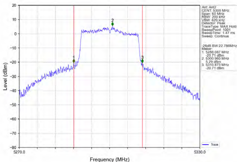
802.11ax(HE20) MCH 5300MHz RU242 Left Ant2 NTN
