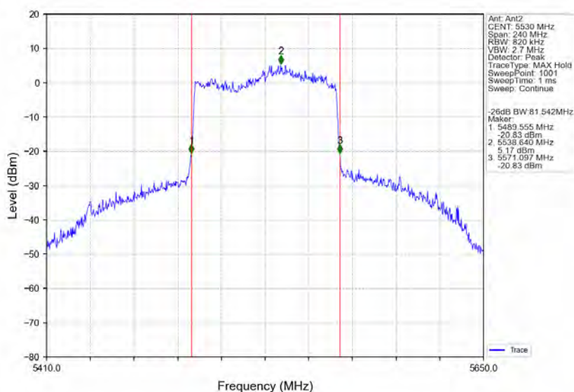
802.11ax(HE80) LCH 5530MHz RU996 Left Ant2 NTNv
