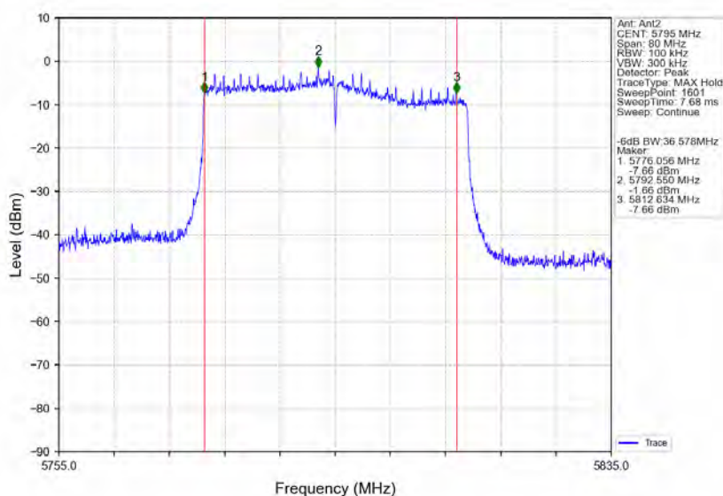
802.11ax(HE40) HCH 5795MHz RU484 Left Ant2 NTNv
