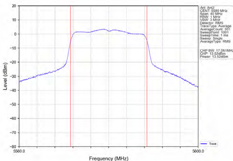
802.11a_MCH_5580MHz_Ant2_NTNV
