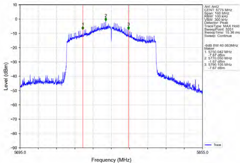
802.11ax(HE80) MCH 5775MHz RU996 Left Ant2 NTN
