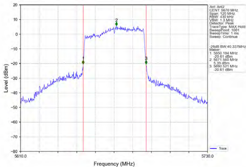
802.11ax(HE40) HCH 5670MHz RU484 Left Ant2 NTNv
