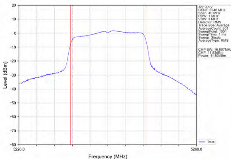
802.11a_HCH_5240MHz_Ant2_NTNV
