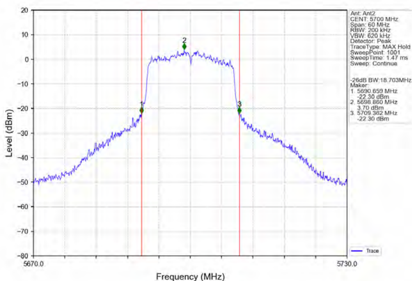
802.11a_HCH_5700MHz_Ant2_NTNV
