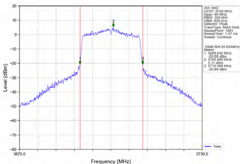
802.11ax(HE20) HCH 5700MHz RU242 Left Ant2 NTNv
