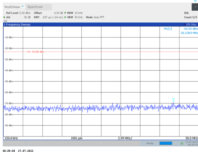
Band26-5MHz-QPSK-26715-1RB#0-Range2:0.15~30MHz
