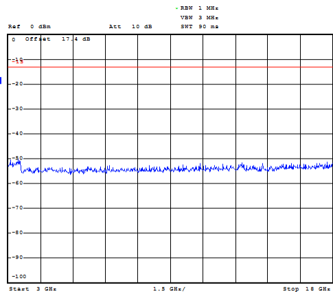
WCDMA Band IV CH-Middle 3GHz~18GHz
