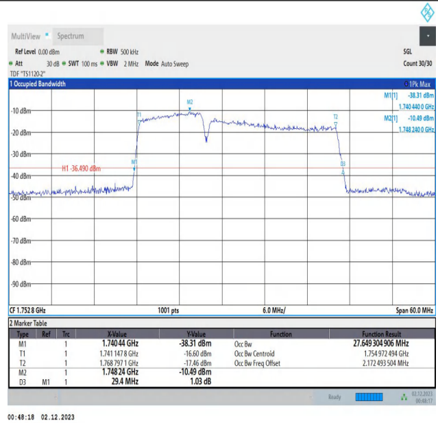
66-66-10MHz-20MHz-QPSK-QPSK-132328-132472-50RB#0 -100RB#0-PASS
