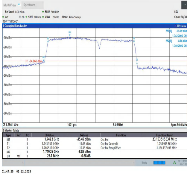
66-66-15MHz-10MHz-QPSK-QPSK-132373-132493-75RB#0 -50RB#0-PASS
