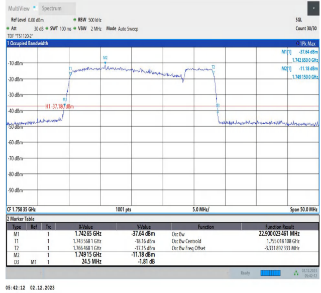
66-66-20MHz-5MHz-QPSK-QPSK-132397-132514-100RB#0 -25RB#0-PASS
