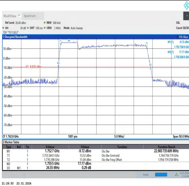
66-66-5MHz-20MHz-QPSK-QPSK-132428-132572-25RB#0- 100RB#0-PASS
