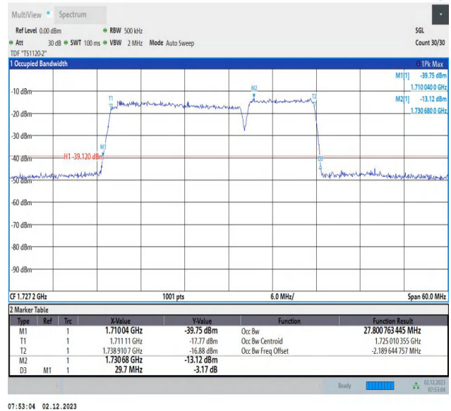
66-66-20MHz-10MHz-QPSK-QPSK-132072-132216-100RB# 0-50RB#0-PASS
