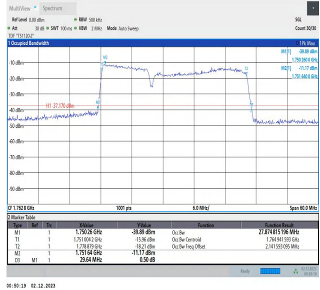
66-66-10MHz-20MHz-QPSK-QPSK-132428-132572-50RB#0 -100RB#0-PASS
