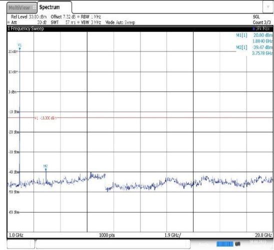
Band25-10MHz-QPSK-26365-1RB#0- Range2:1000~20000MHz
