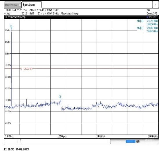
Band25-20MHz-QPSK-26590-1RB#0- Range2:1000~20000MHz
