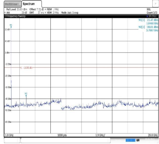
Band25-15MHz-QPSK-26115-1RB#0- Range2:1000~20000MHz
