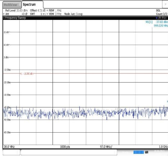
Band25-10MHz-QPSK-26365-1RB#0- Range1:30~1000MHz
