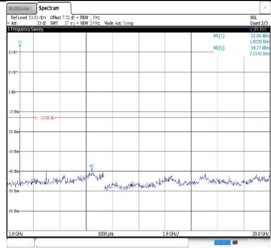
Band25-3MHz-QPSK-26055-1RB#0- Range2:1000~20000MHz
