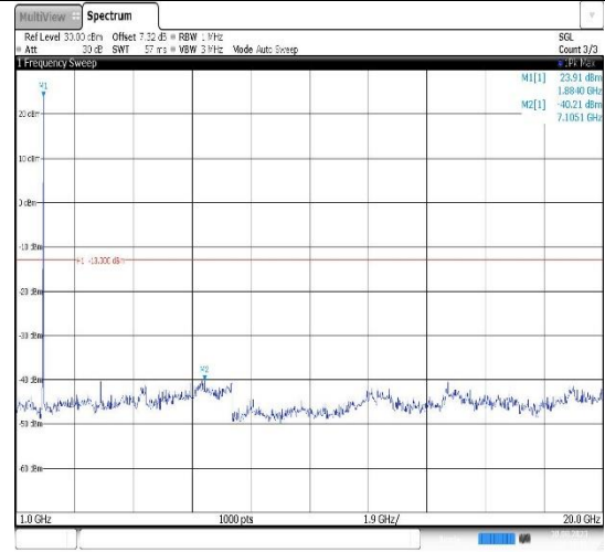
Band25-15MHz-QPSK-26365-1RB#0- Range2:1000~20000MHz
