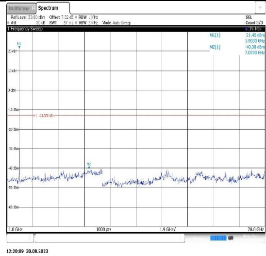
Band25-20MHz-QPSK-26140-1RB#0- Range2:1000~20000MHz
