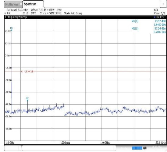
Band25-5MHz-QPSK-26065-1RB#0- Range2:1000~20000MHz
