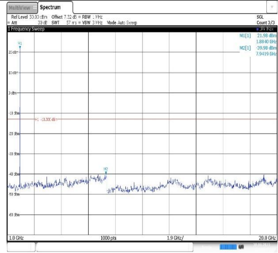
Band25-10MHz-16QAM-26365-1RB#0- Range2:1000~20000MHz
