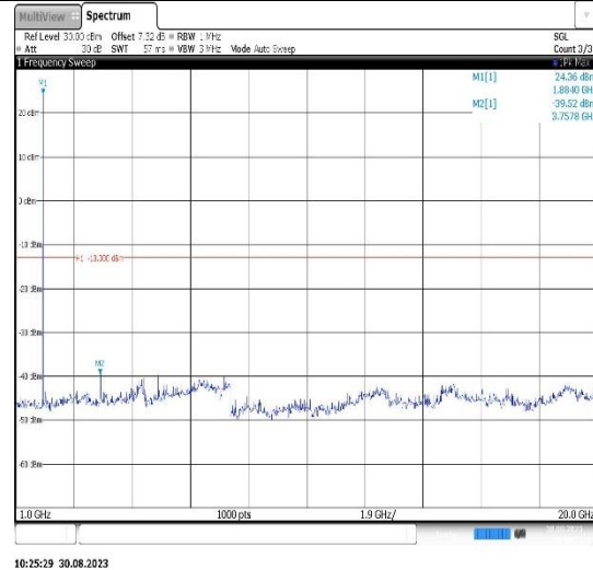
Band25-1.4MHz-QPSK-26683-1RB#0- Range2:1000~20000MHz
