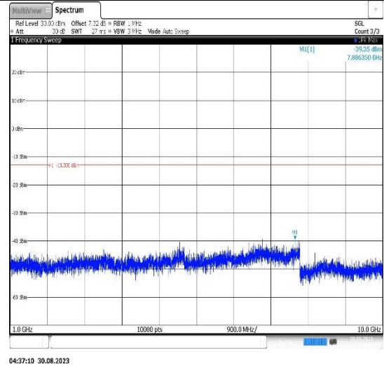
Band12-10MHz-QPSK-23130-1RB#0- Range2:1000~10000MHz
