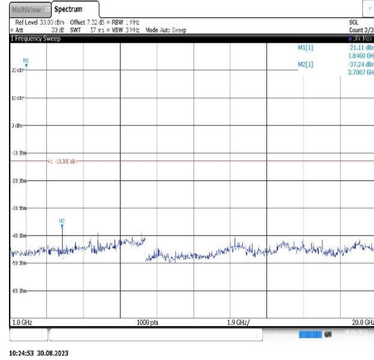
Band25-1.4MHz-QPSK-26365-1RB#0- Range2:1000~20000MHz
