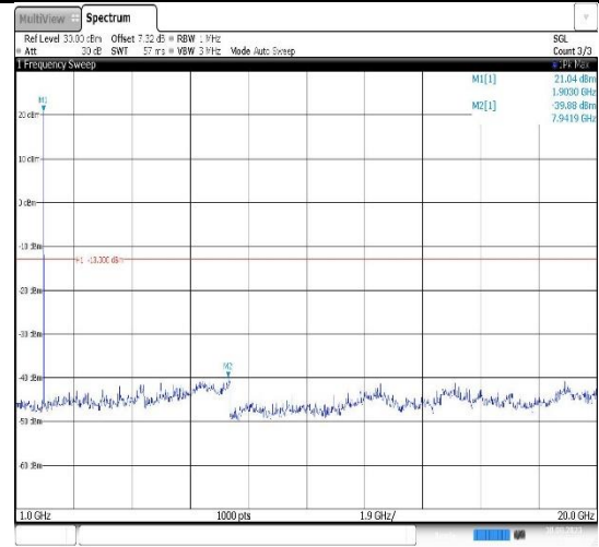
Band25-10MHz-QPSK-26090-1RB#0- Range2:1000~20000MHz
