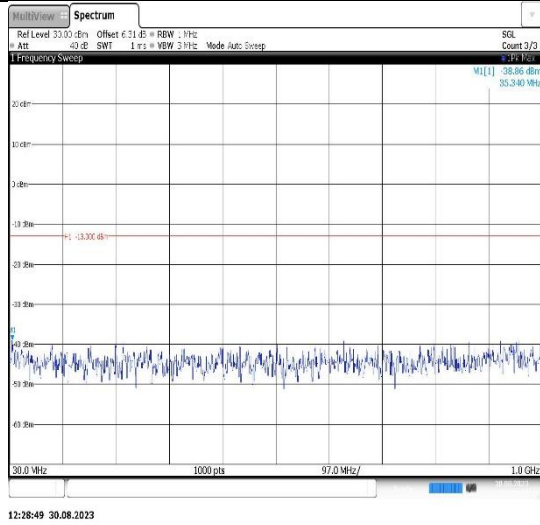
Band25-20MHz-QPSK-26365-1RB#0- Range1:30~1000MHz
