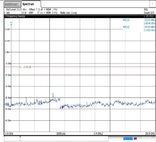
Band25-5MHz-QPSK-26365-1RB#0- Range2:1000~20000MHz
