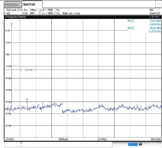
Band25-3MHz-QPSK-26365-1RB#0- Range2:1000~20000MHz
