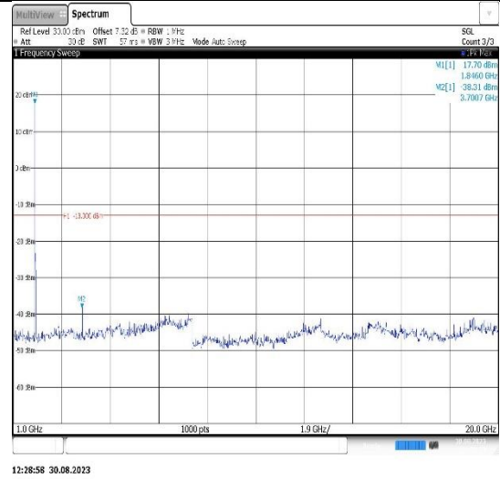
Band25-20MHz-QPSK-26365-1RB#0- Range2:1000~20000MHz
