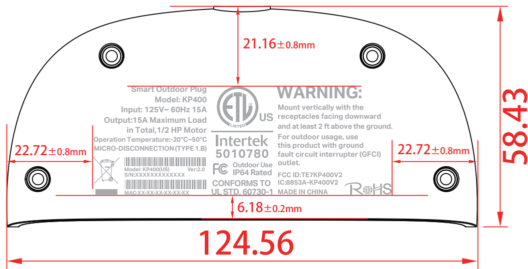
尺寸图
