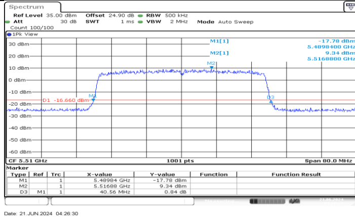
11AX40MIMO_Ant4_5510
