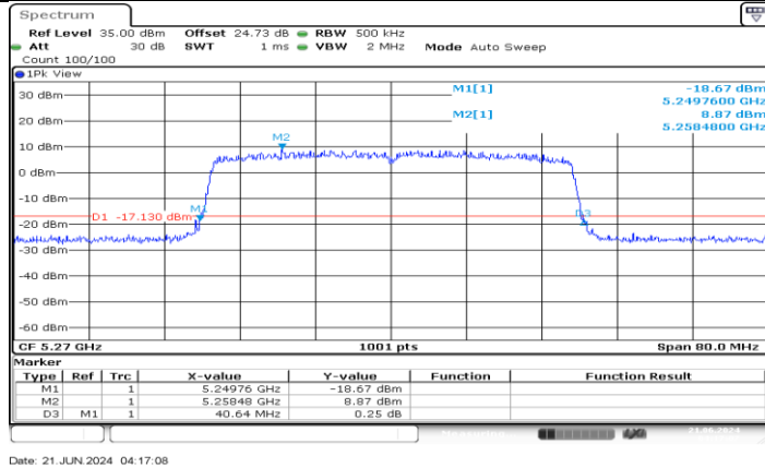
11AX40MIMO_Ant3_5270
