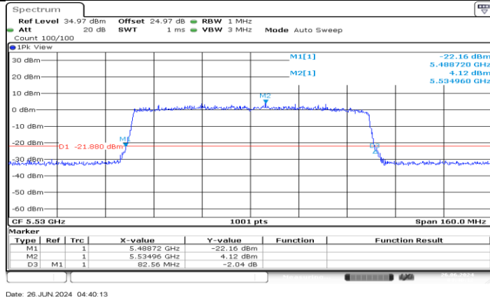
11AX80MIMO_Ant3_5530
