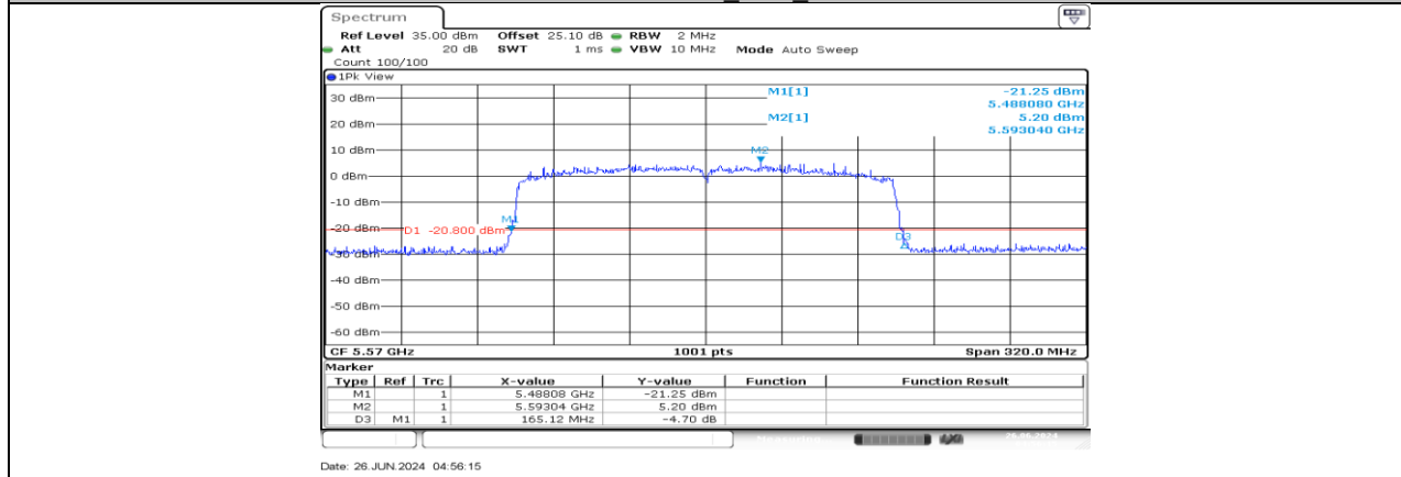
11AX160MIMO_Ant4_5570
