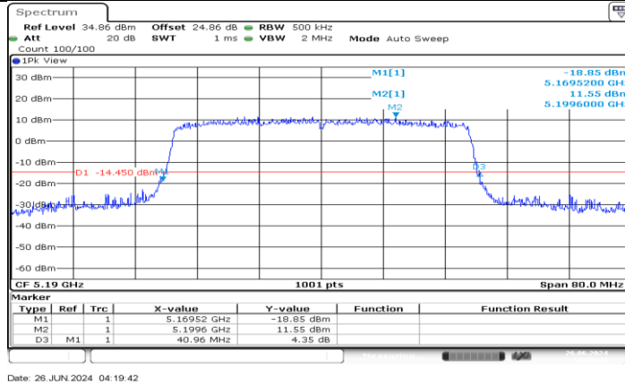
11AX40MIMO_Ant4_5190
