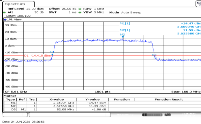
11AX80MIMO_Ant4_5610
