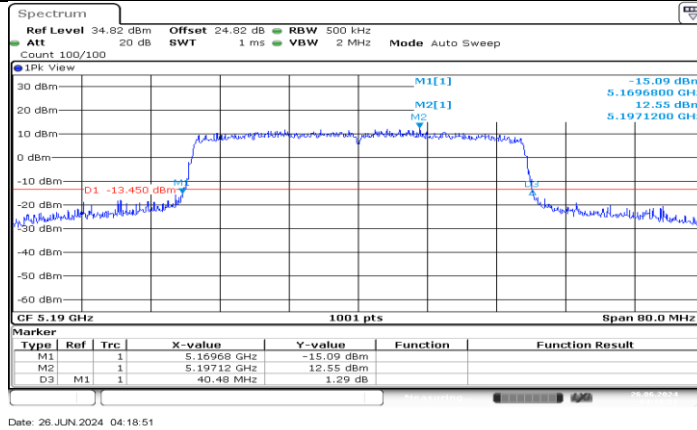
11AX40MIMO_Ant3_5190
