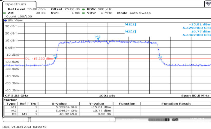
11AX40MIMO_Ant3_5550
