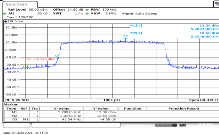
11AX40MIMO_Ant1_5230
