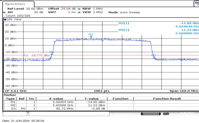
11AX80MIMO_Ant3_5610
