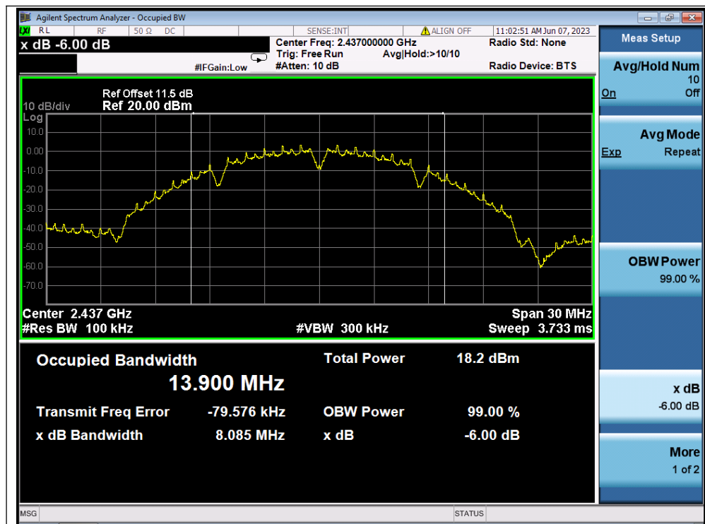
(Channel 6, 802.11b)
