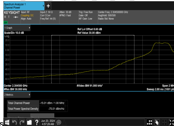
B2_N30(5M)_DFT-s- OFDM_QPSK_Edge_1RB_Left_Low_CH_CHP_PAS
