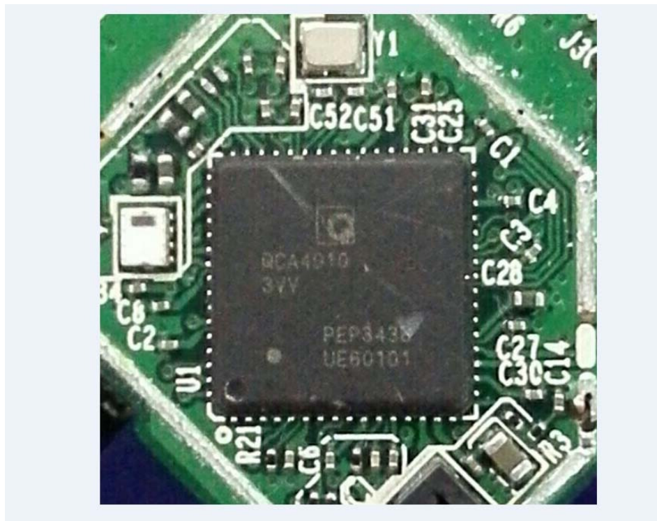
(6) EUT Photo
