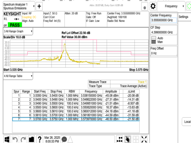
Band48_10MHz_CP_OFDM_SCS30kHz_QPSK_RB1_23_CH637000
