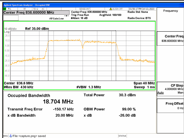
5B / 10+10MHz / 64QAM/ Mid CH
