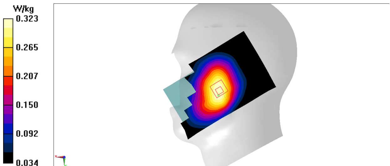
Fig.5 WCDMA 850
